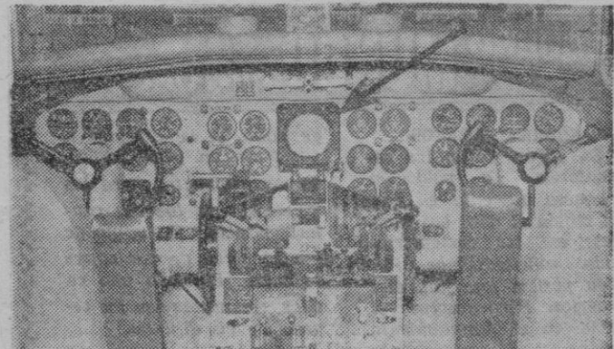
Mamparo de mandos del «Metropolitan». En el centro, señalado por la flecha, la pantalla del «radar». —(Foto Mario)
