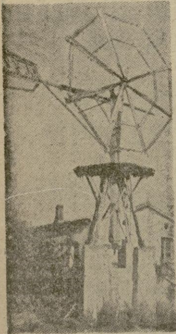
Molino y caballete de madera, de la serie de los trazados por Damián Reixach.
