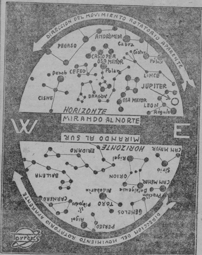
ASPECTO DEL CIELO EL DIA 1 DE ENERO A LAS 22 HORAS (HORA OFICIAL) CON LAS PRINCIPALES CONSTELACIONES Y PLANETAS FACILMENTE OBSERVABLES.
