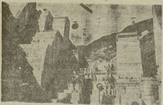
Fase de colocación de las tuberías de toma. Los seis blindados o especiales grúas aéreas están aquí en plena actividad, en las obras de construcción de la presa del salto de Salime (8 de mayo 1952).
