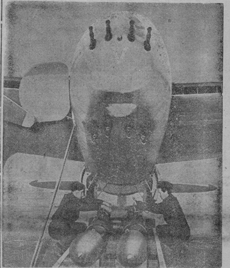
El «Mosquito» es un tipo de bombardero ligero y de aparato de batalla de la R.A.F. que ha dado un excelente resultado. Aquí vemos a uno de ellos de frente repostando gasolina.
