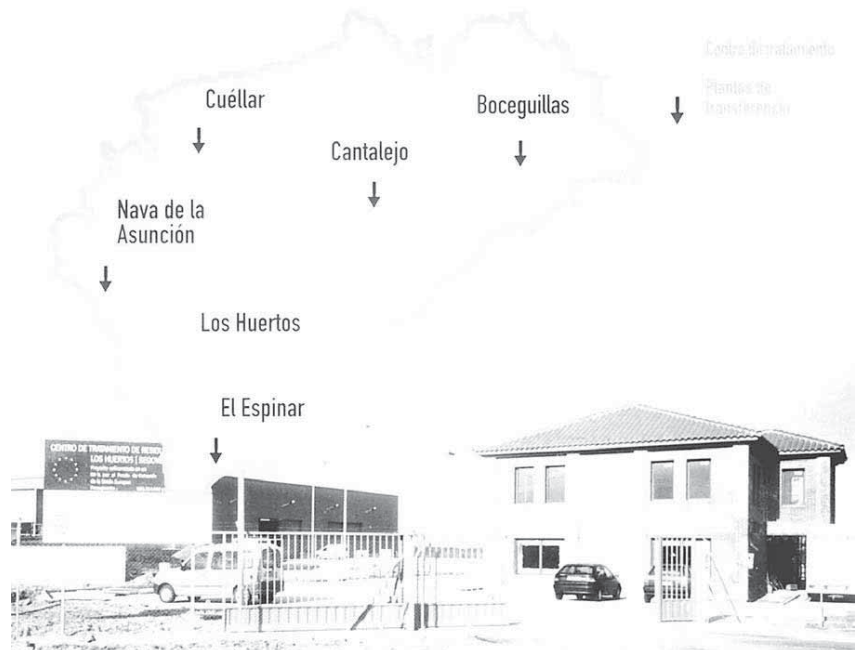
El sistema de gestión de R.S.U. de Segovia se basa en gran parte en un centro de tratamiento y cinco plantas de transferencia
