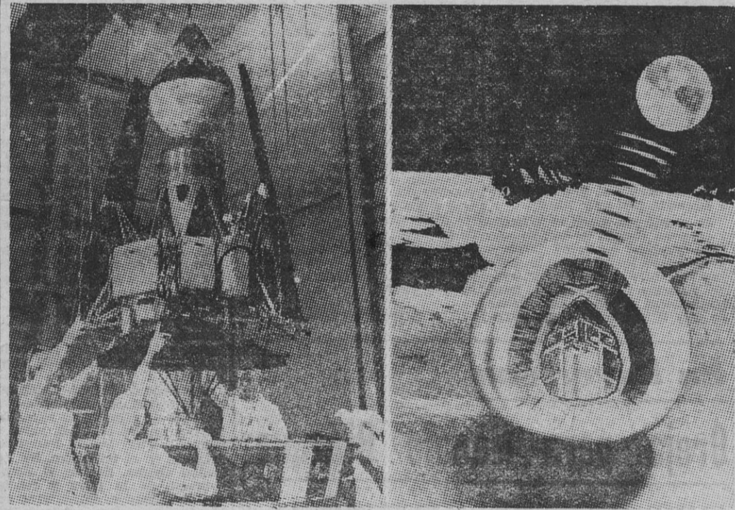
Un grupo de técnicos examinan, a la izquierda, la nave espacial «Ranger V», preparada para su lanzamiento mañana, desde Cabo Cañaveral, con destino a la Luna. En su parte superior lleva una esfera cubierta de madera de balsa, destinada a ser depositada sobre la superficie lunar. Los instrumentos dispuestos en el interior de esta cápsula, a la derecha, registrarán los temblores lunares, o «lunamotos», los impactos de meteoritos y las temperaturas, cuyas mediciones serán enviadas por radio a la Tierra durante un mes.
