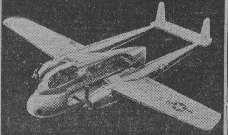
Así interpreta un artista el nuevo avión norteamericano de transporte, el "XC-120", que se dispone a realizar su primer vuelo en Hagerstown, Maryland. La distribución está realizada de tal forma que puede descargarse en cualquier aeropuerto su fuselaje, con pasajeros y carga, y despegar con otro fuselaje. — (Foto Cifra)
