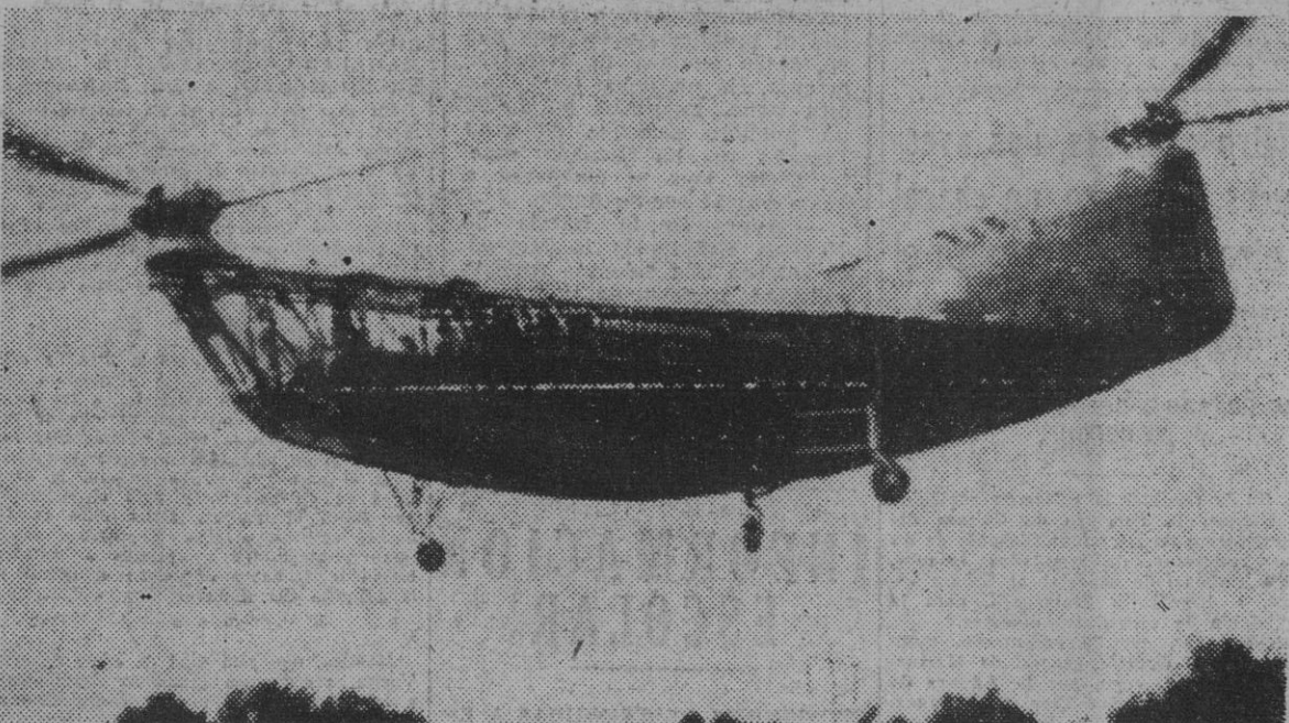
Proyectado para la Marina y para las escuadrillas de salvamento del servicio de guardacostas de los Estados Unidos, el nuevo helicóptero "PV-3", el mayor aparato de este tipo del mundo, efectúa sus pruebas de vuelo sobre el campo de las fábricas de Sharen Hill (Foto Sena, recibida por radio)
