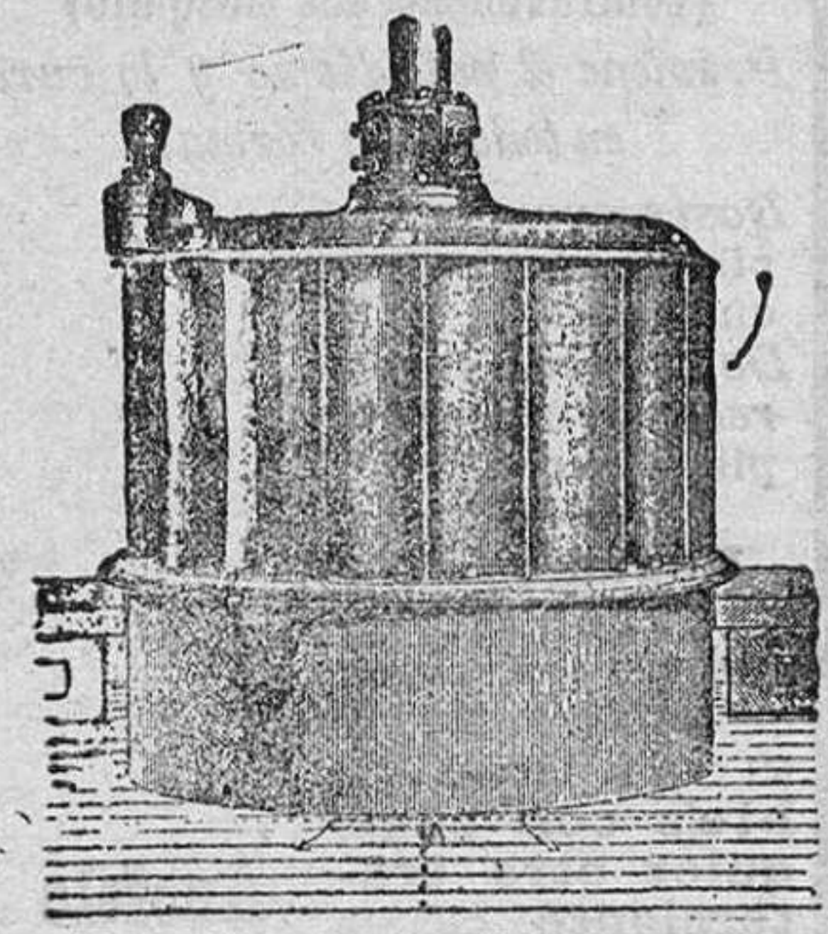
Turbina americana.
