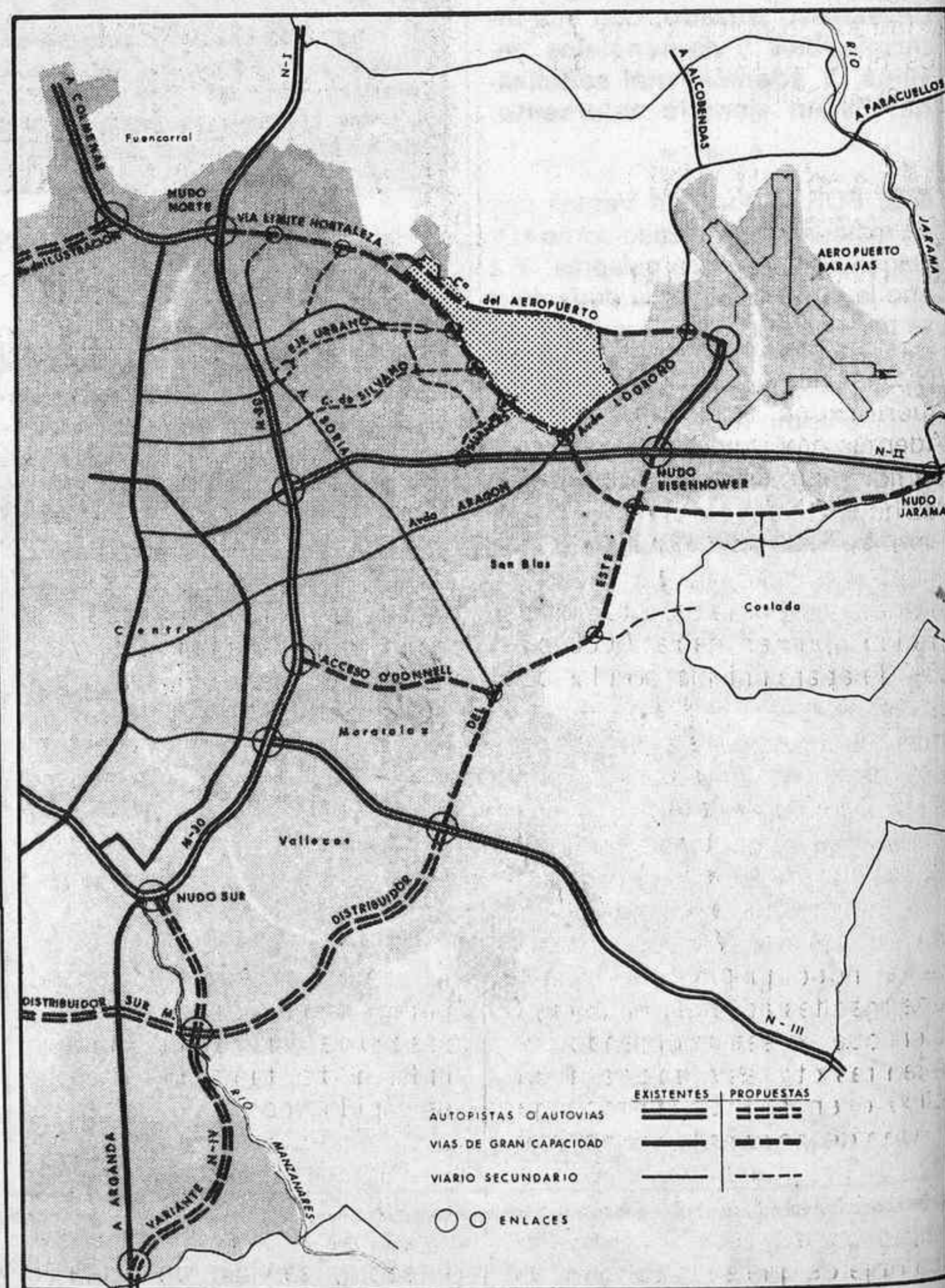
Esquema de los accesos al recinto ferial, los ya existentes y los que ya están propuestos para su construcción.
