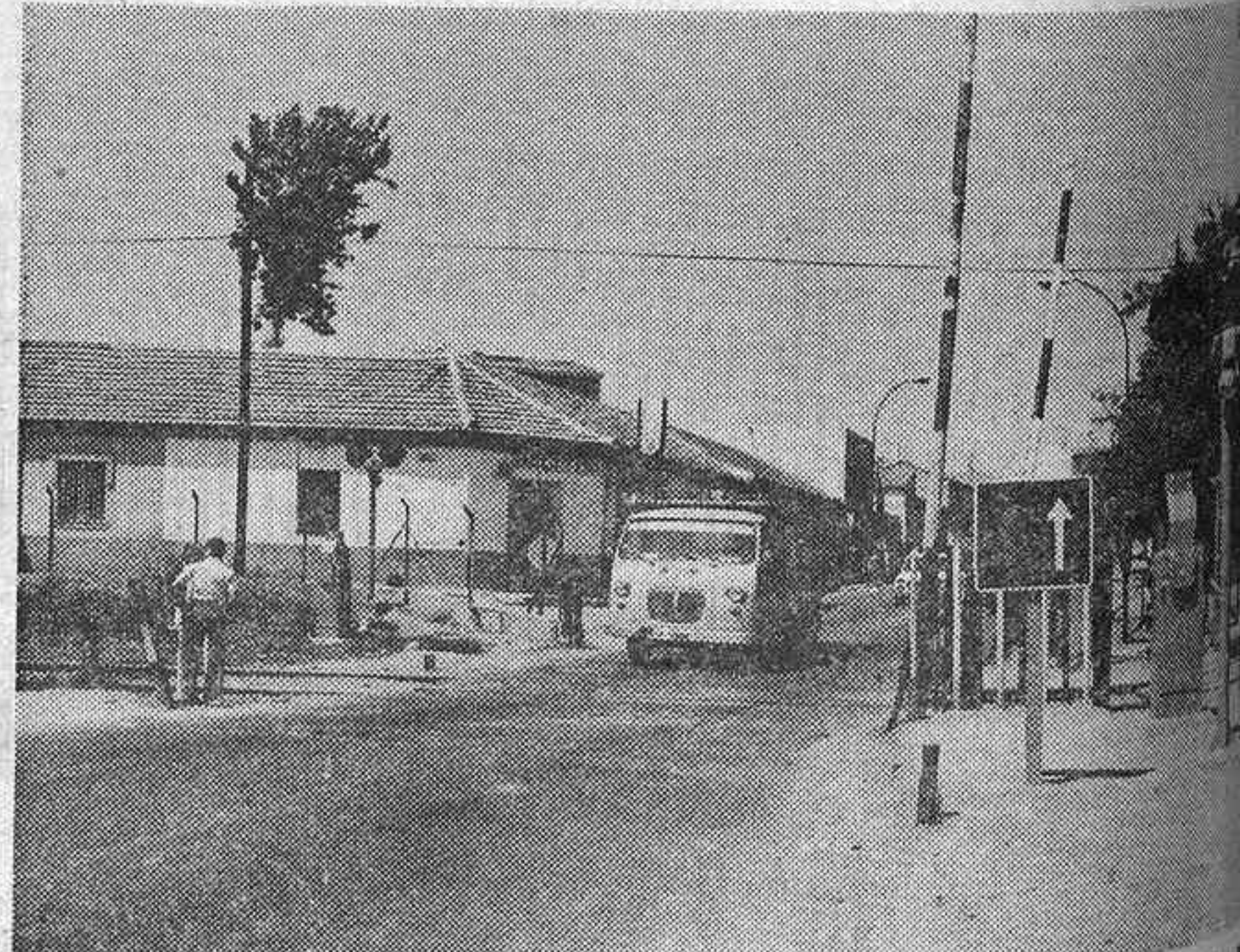
Para la construcción de los pasos a nivel han sido cumplidas las condiciones que imponen. Concretamente el de Leganés tendrá unas características especiales por la configuración de la vía descendente de 7,4 por 100. (Foto Torremocha.)
