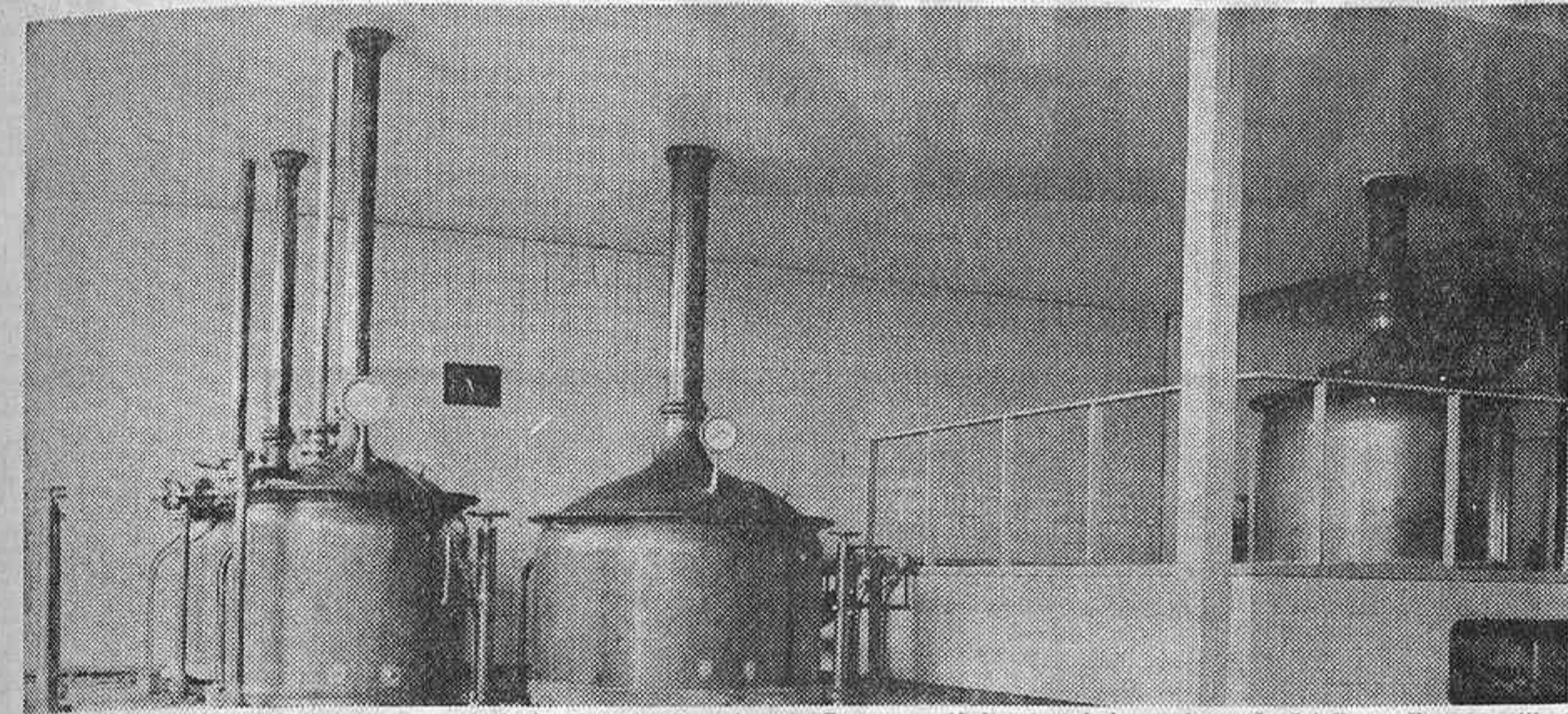
Sala de cocción de la fábrica de cerveza de la Escuela Superior de Cerveza y Malta, instalada en Arganda del Rey. (Foto Portillo.)
