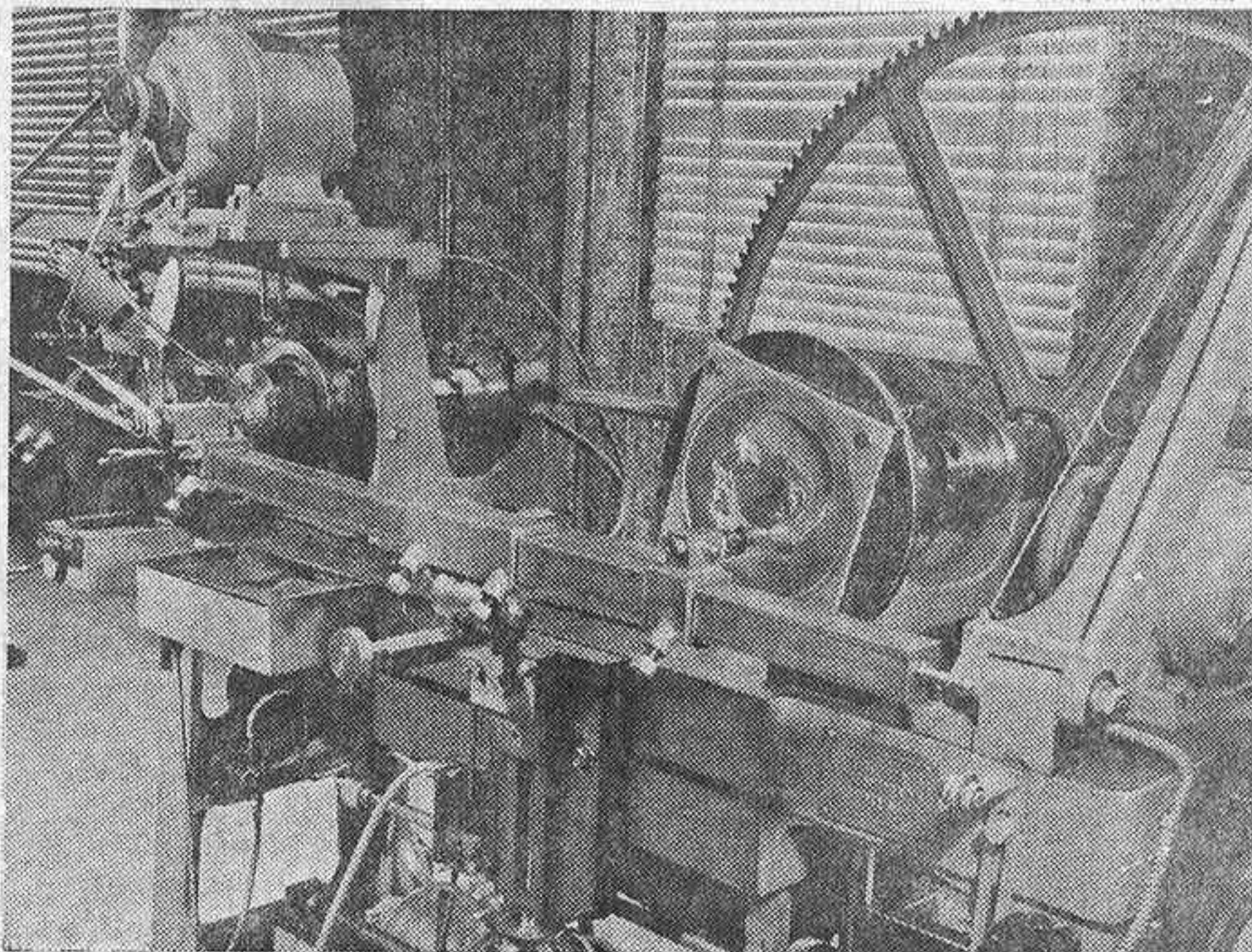
Una máquina de la fábrica de la Moncloa, en acción
