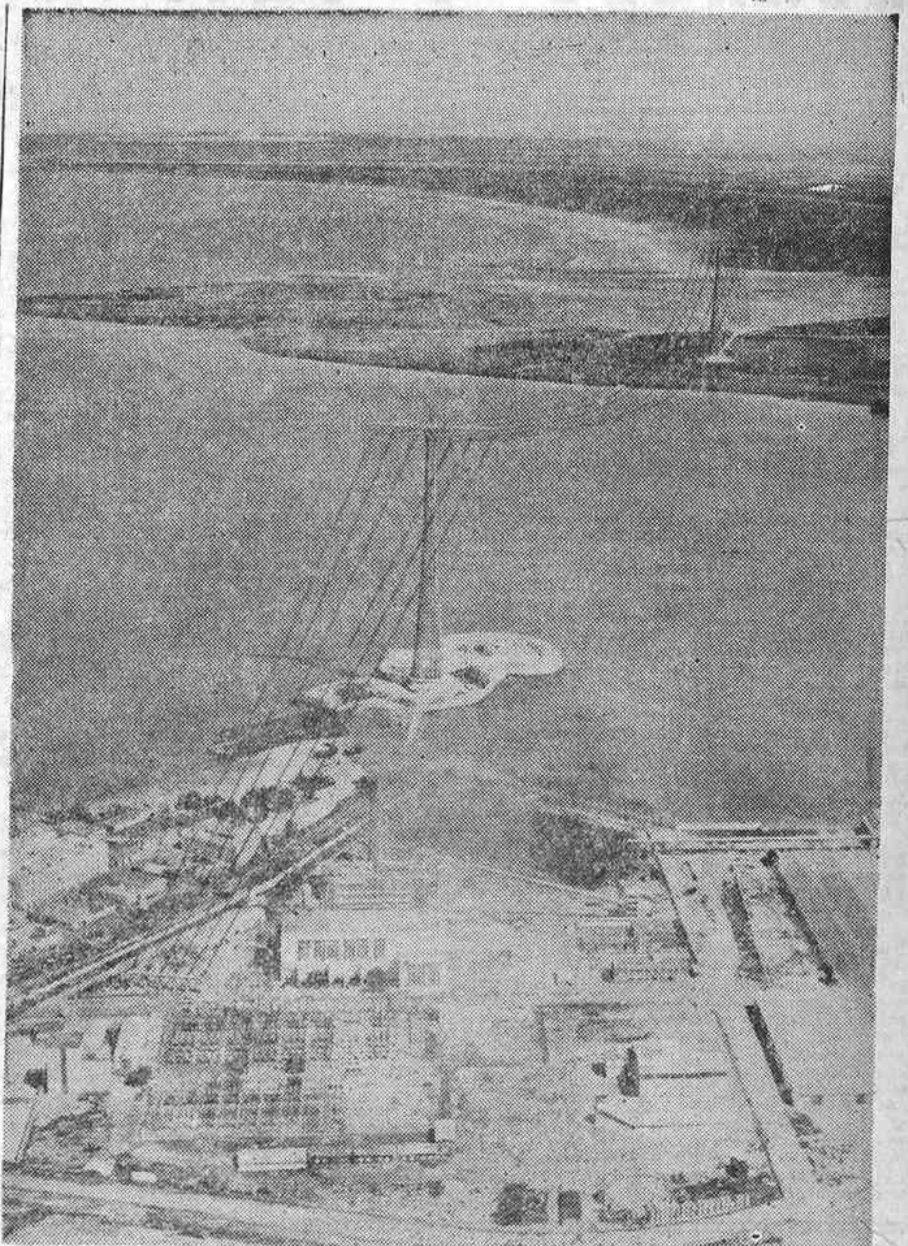
Vista de las dos enormes torres metálicas instaladas en la bahía de Cádiz para la conducción de la energía eléctrica
