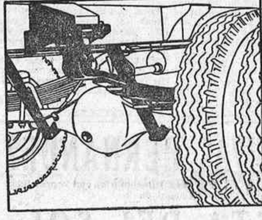
PUNTE TRASERO Punte trasero con pilón de ataque guiado a sus dos extremos por cojinetes cónicos. Palieres flotantes.
