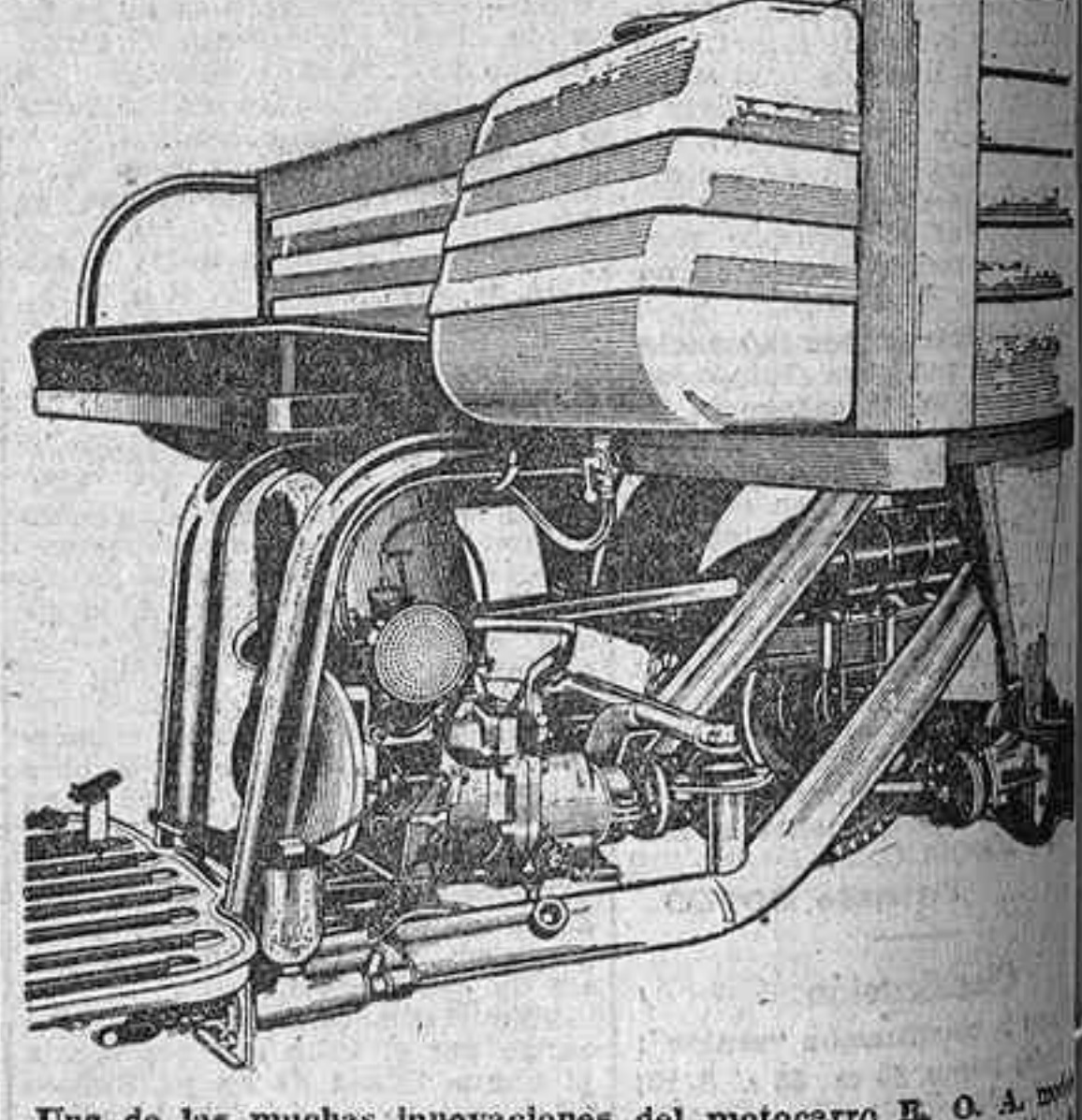
Una de las muchas innovaciones del motocarro R. O. A. modelo R. C. 600: el motor flotante. Algo definitivo en esta clase de vehículos de tan óptimos resultados prácticos.
