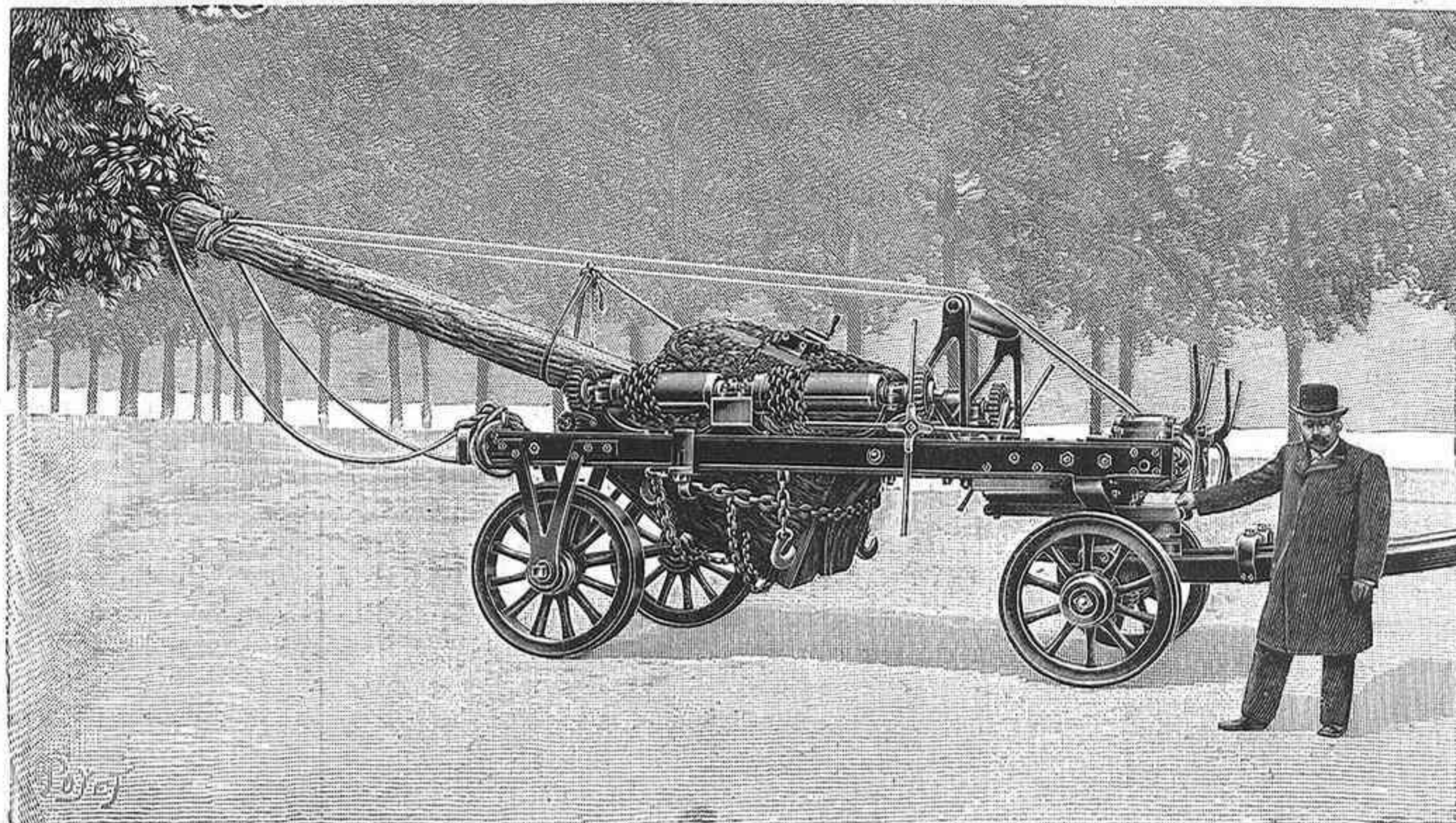
CARRO PARA TRANSPORTAR ÁRBOLES. — Vista de conjunto
