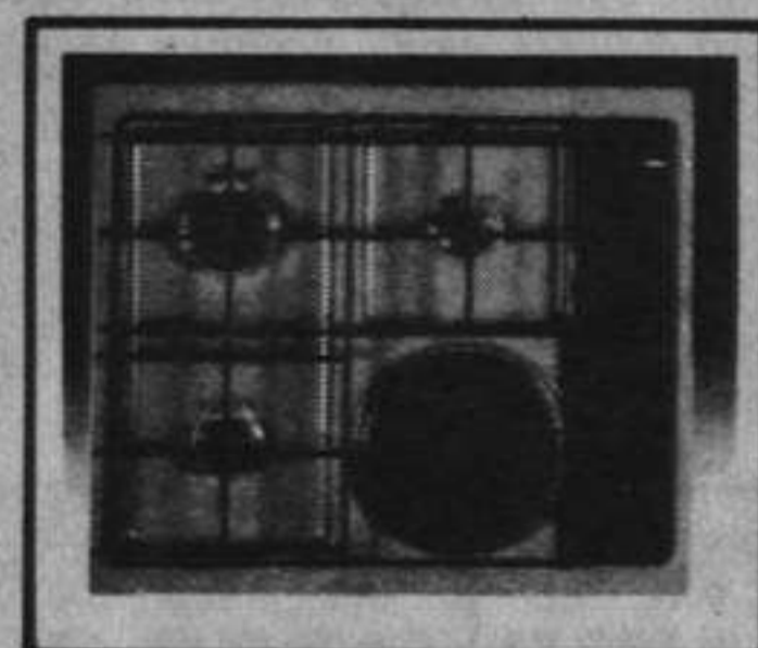
EC/31/E-M Realizadas en chapa esmaltada, con tres fuegos a gas dotados de encendido automático y una placa eléctrica. Zona de mandos serigrafada con un separador que los protege de la zona de combustible. Rejilla de apoyo y tapas de quemadores esmaltadas.
