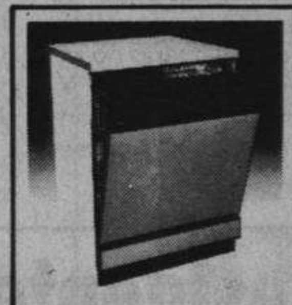
LP/812/PE Piloto indicador de funcionamiento. Piloto indicador de nivel de abrillantador. Descalcificador automático de gran capacidad. Dosificador automático de líquido abrillantador. Dimensiones normalizadas: 85 cm. alto; 59,7 cm. ancho y 60 cm. profundidad.
