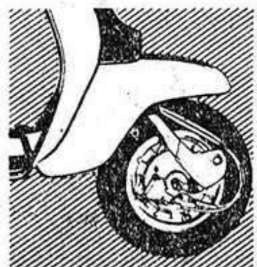
Suspensión perfecta por bielas oscilantes. Amplias superficies de frenado.
