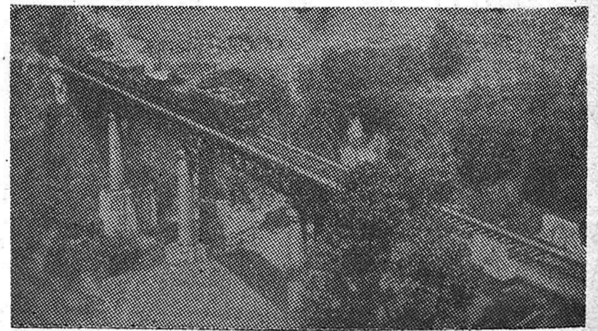
He aquí uno de los trenes eléctricos que prestan servicio en la línea electrificada de Irún, a su paso por el puerto de Pasajes, cerca de San Sebastián. Al lado de velocidad se ganó limpieza: la carbonilla ha desaparecido.
