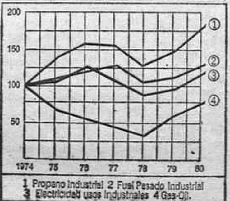
PRECIO PRODUCTOS ENERGETICOS INDUSTRIALES EN PTAS. CONSTANTES (en forma de números índices)
