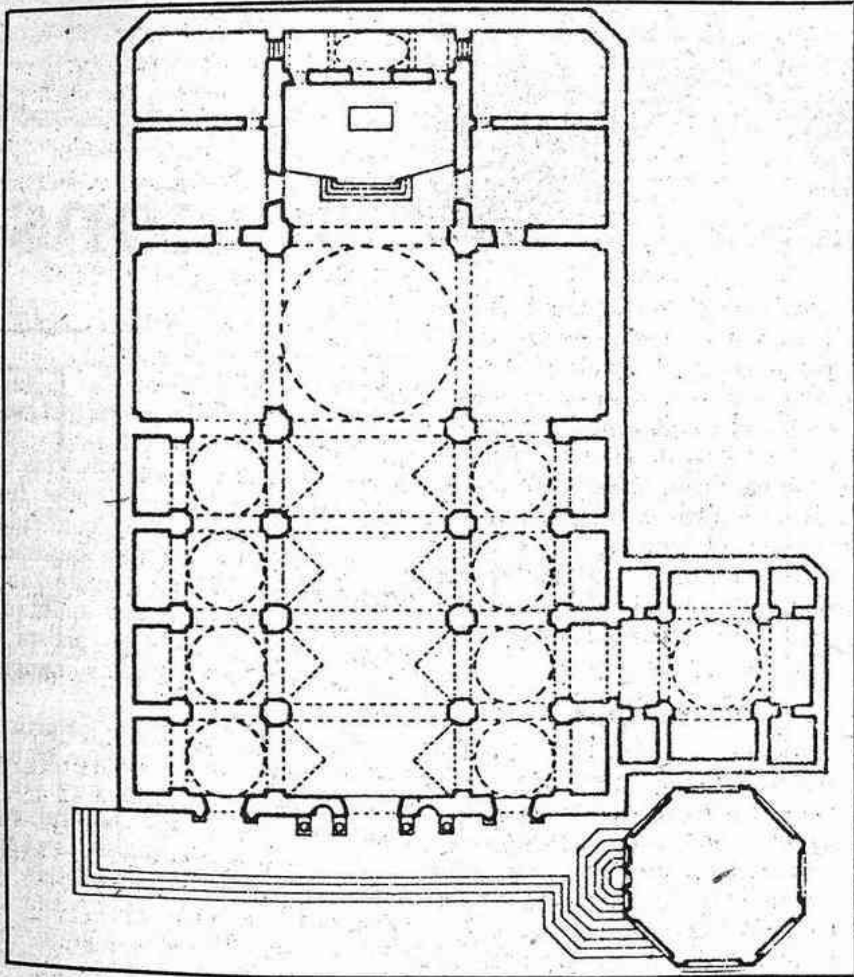
Planta de la iglesia y torre campanario
