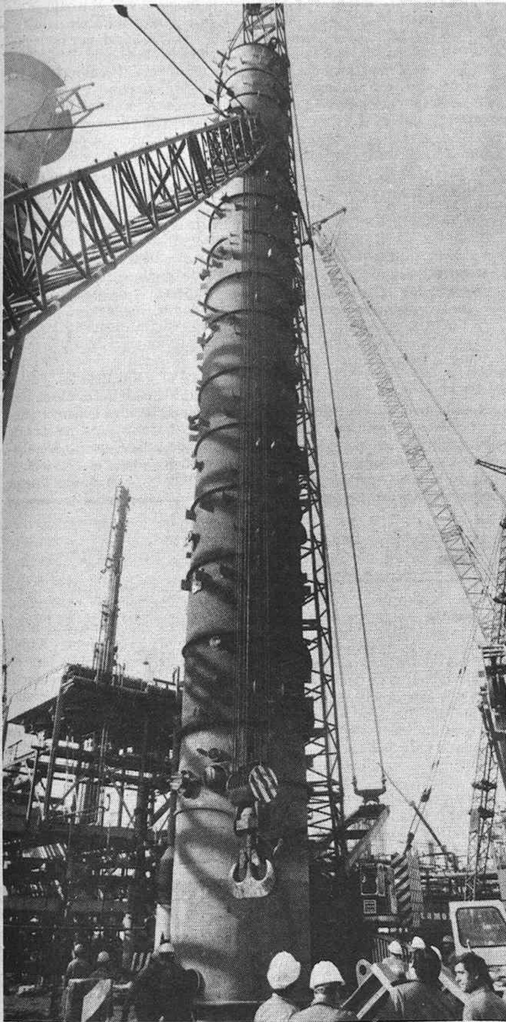
Ayer se montó la torre fraccionadora de la refinería de Petromed
