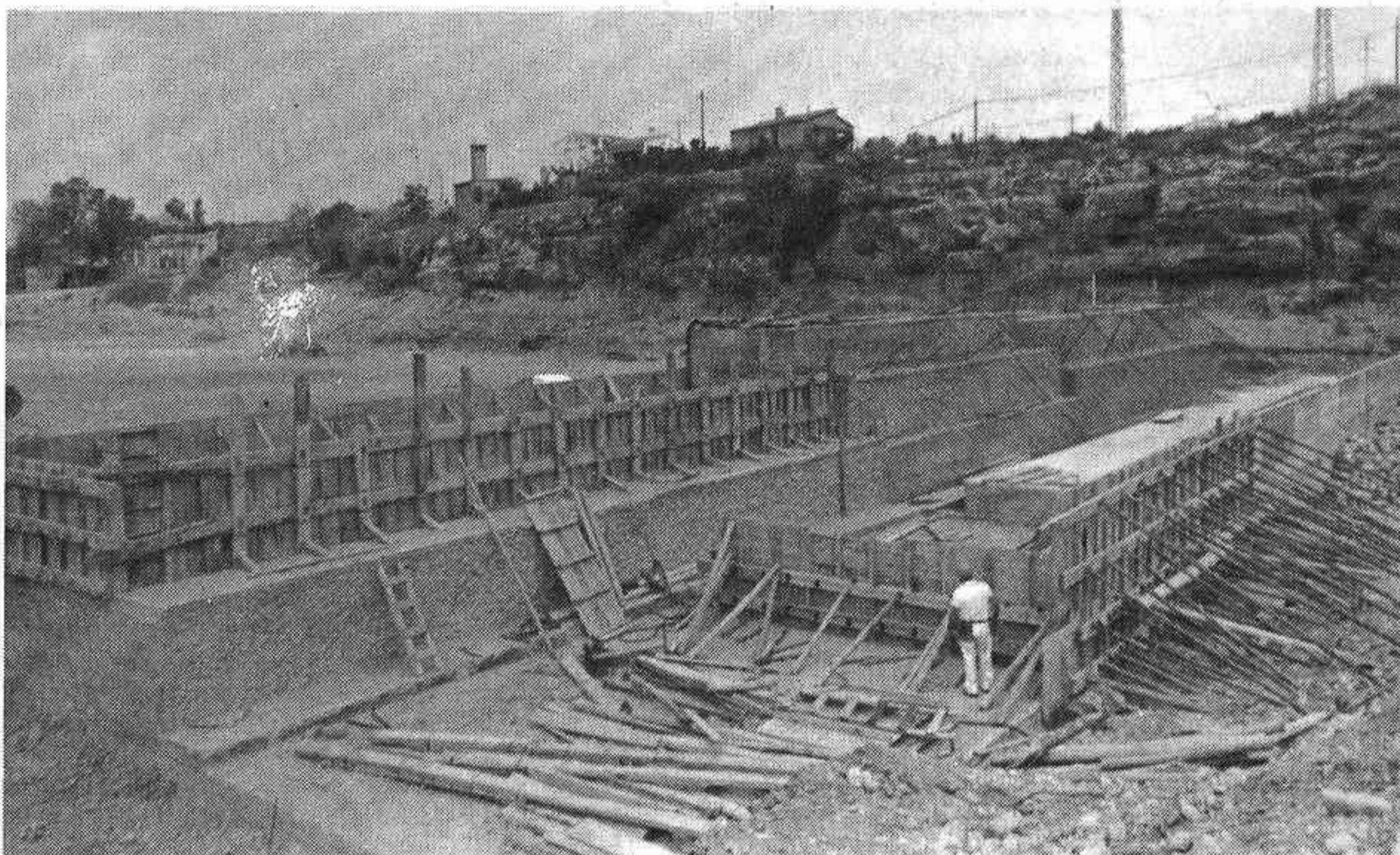
Aspecto general de las obras en el cauce del Mijares
