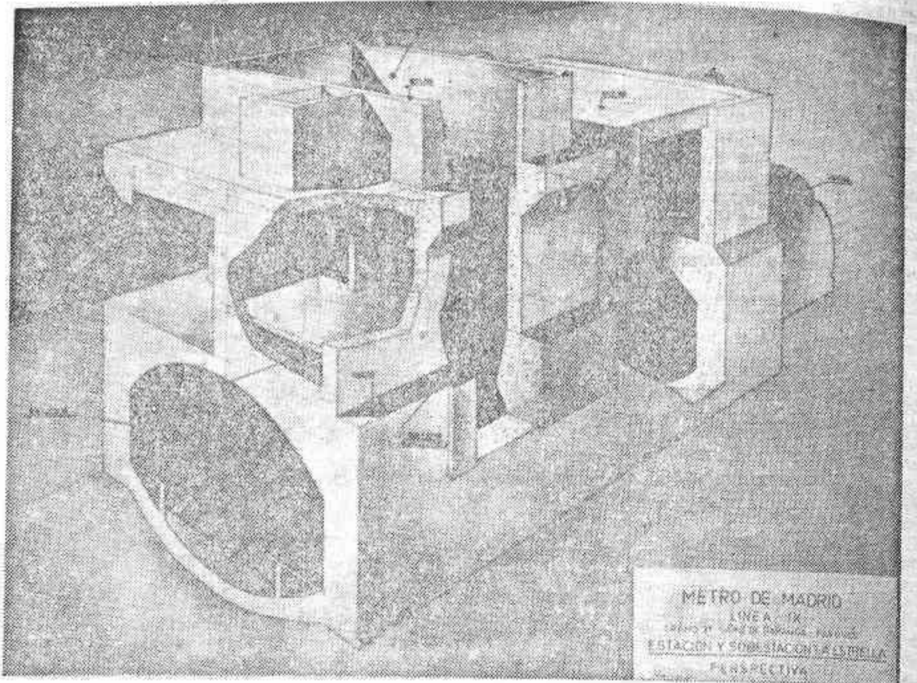
Perspectiva de la estación y subestación la Estrella.
