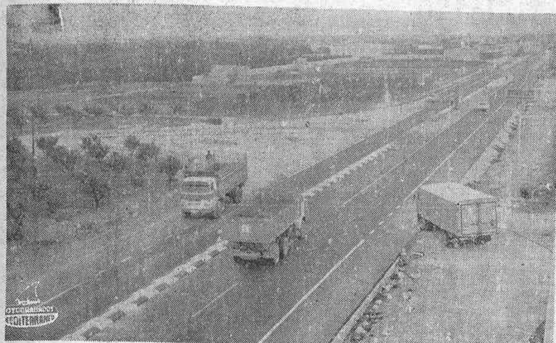
Intersección del acceso de Vinaroz a Ulldecona en la carretera nacional 340
