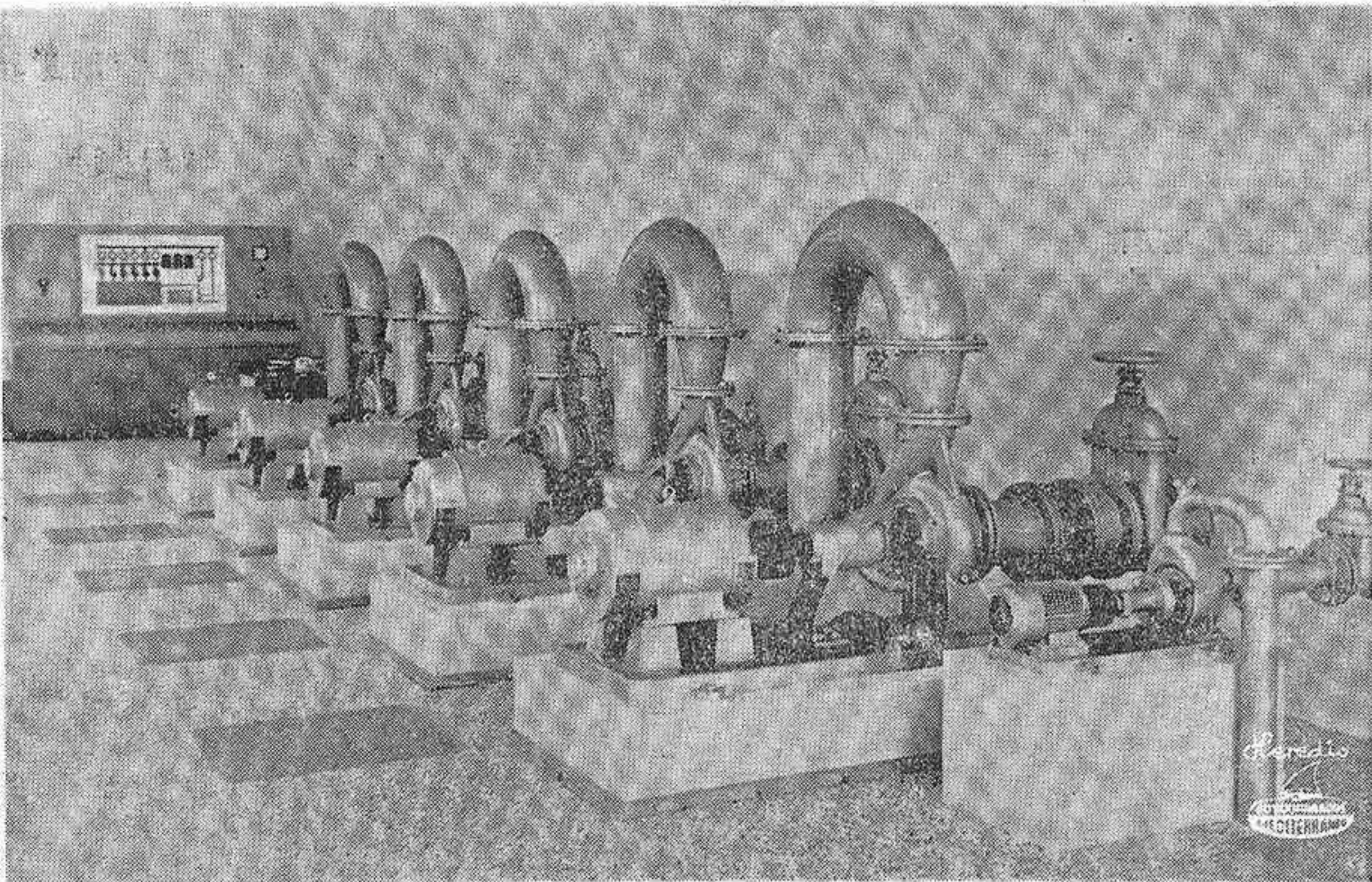
Conjunto de bombas que impulsan el agua, desde el depósito, a la red de distribución
