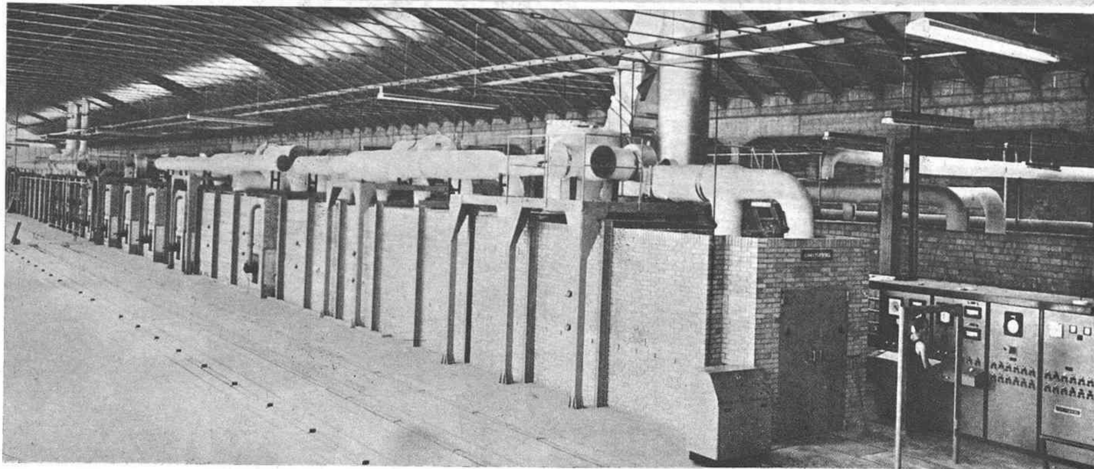
Hornos tunel.es para biscochado y esmaltado
