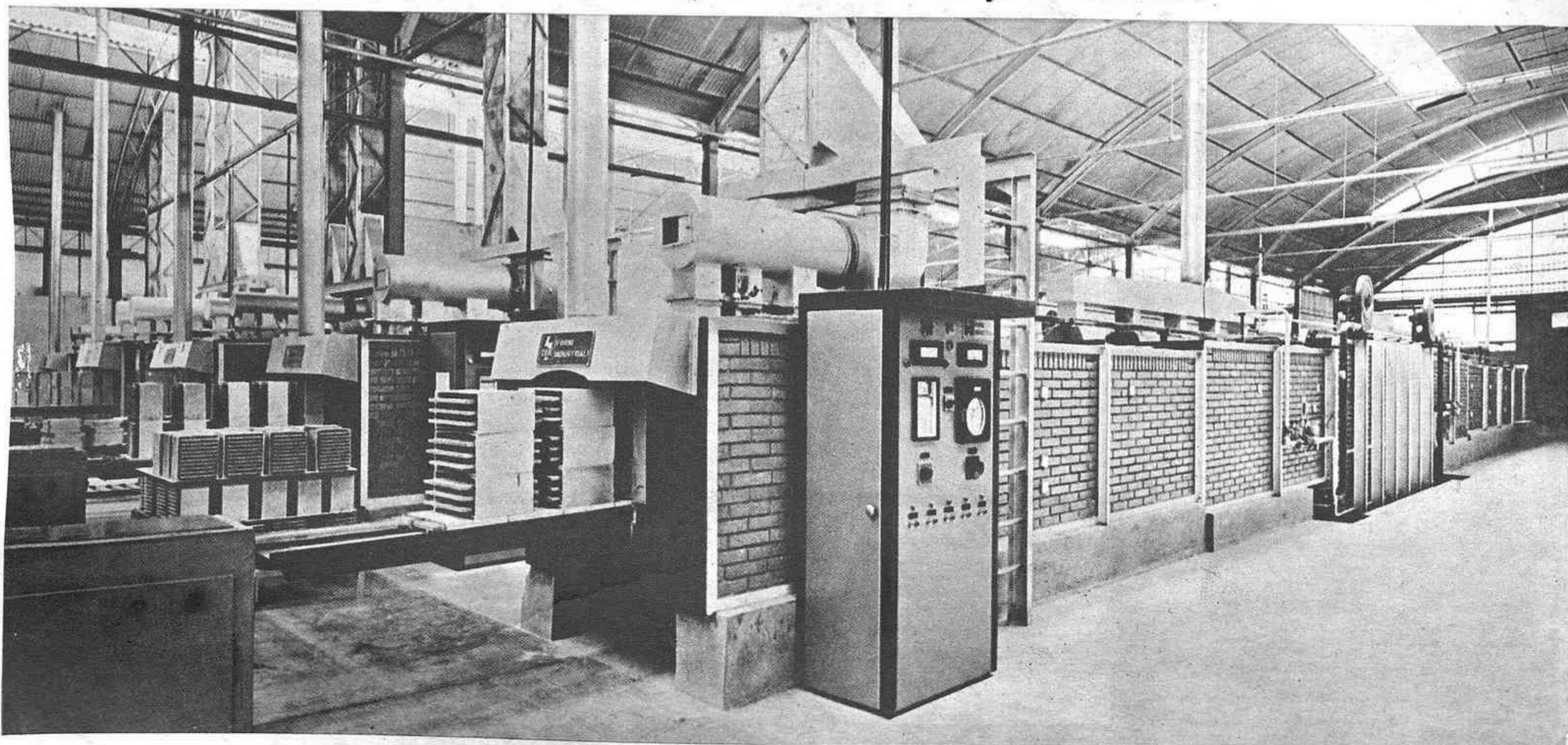
Hornos bicanales para esmaltados
