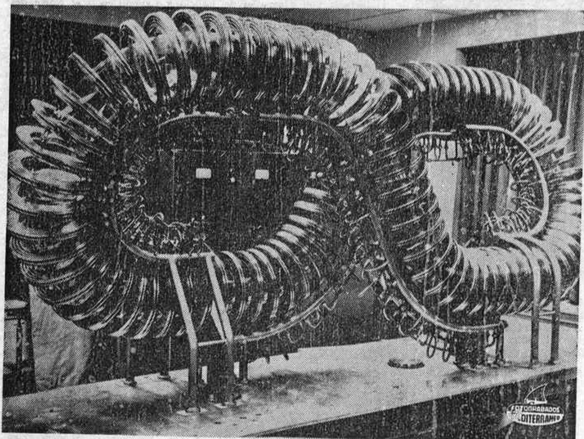
Un ingenioso dispositivo en forma de ocho que sirve para almacenar hidrógeno a temperaturas elevadísimas y estudiar las posibilidades de utilizar comercialmente el fenómeno de fusión nuclear.
