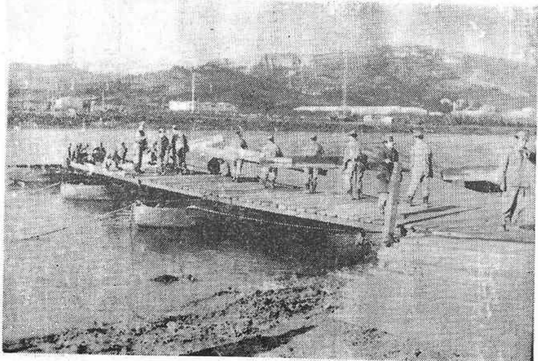
MOLINS DE REY. — Una vista general de los trabajos de instalación por parte del Ejército, de un paso militar sobre el río Llobregat, para normalizar el paso de peatones en ambas orillas. — (Telefoto Cifra Grafica).
