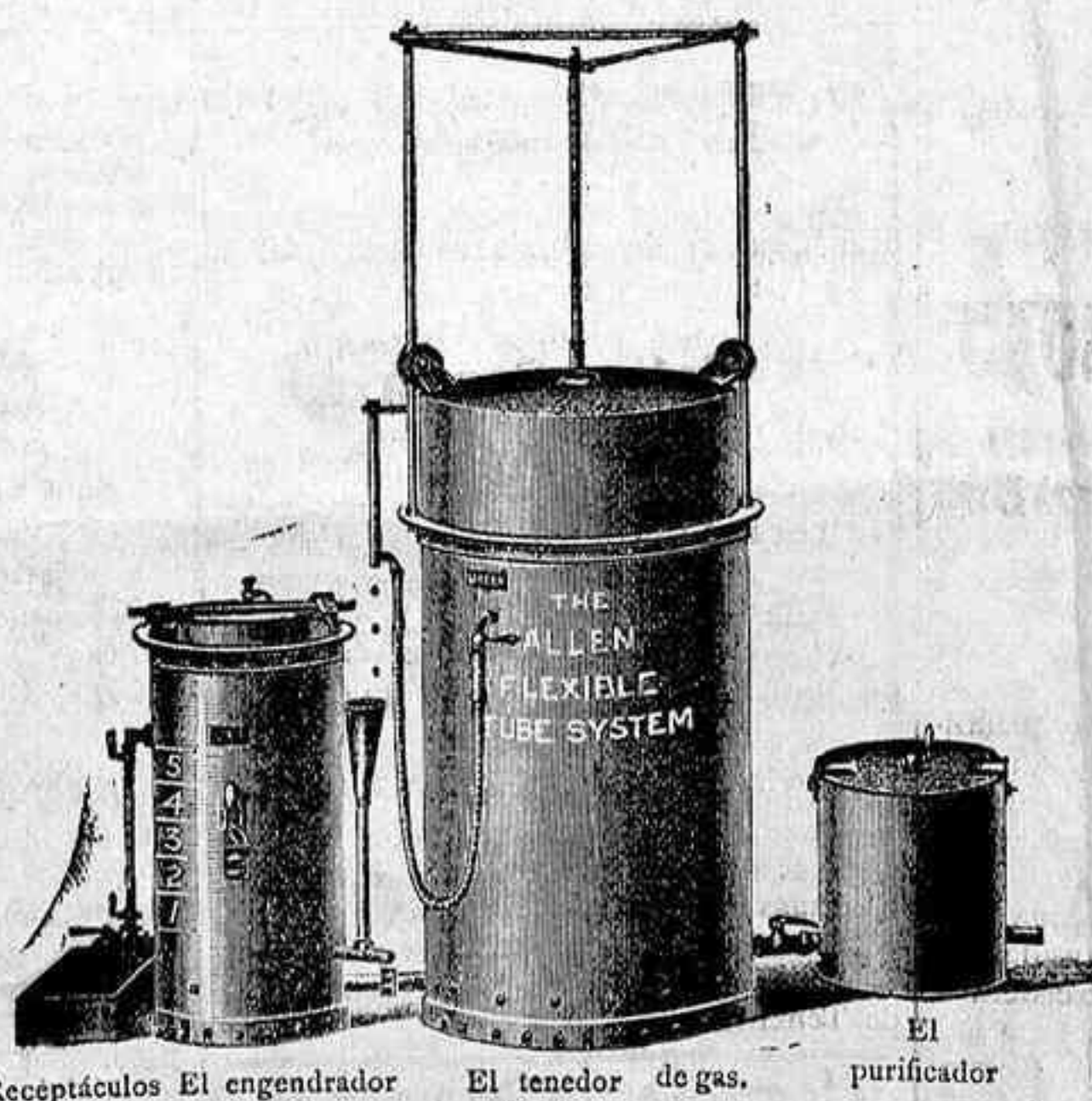
Receptáculo de "carbido"
