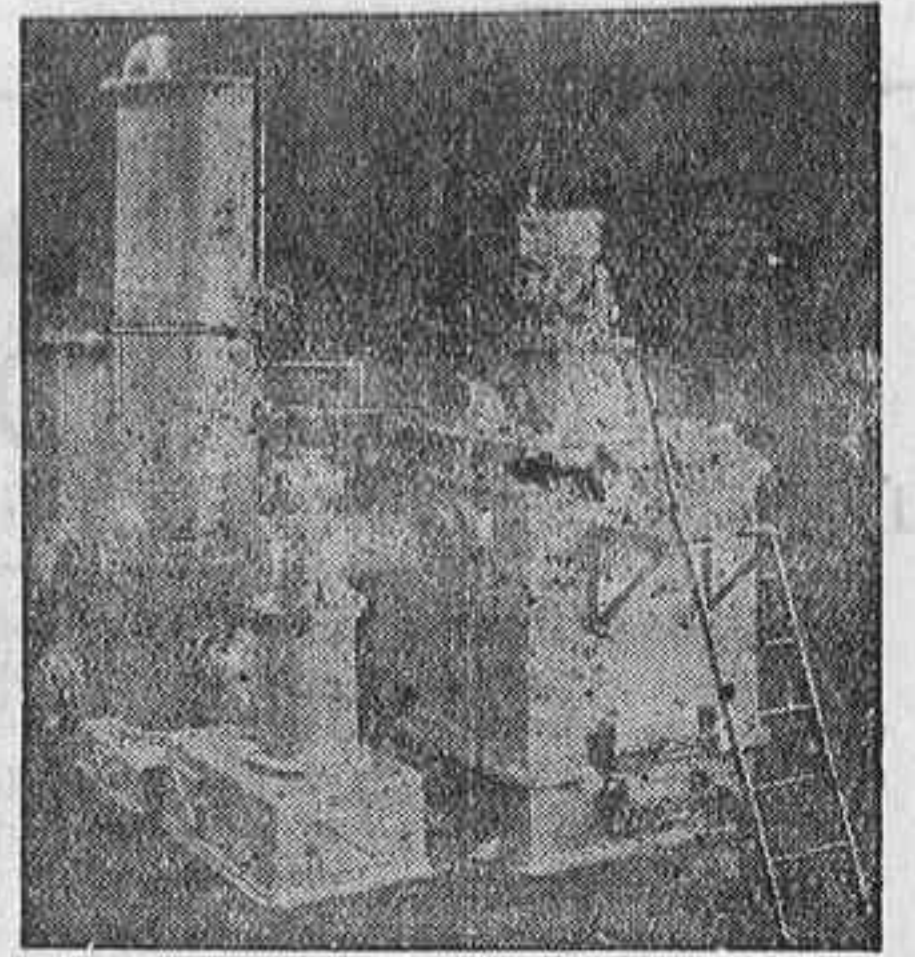
Gasógeno sencillo
