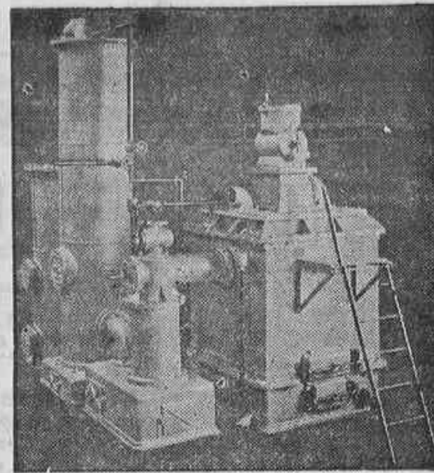
Gasógeno sencillo
