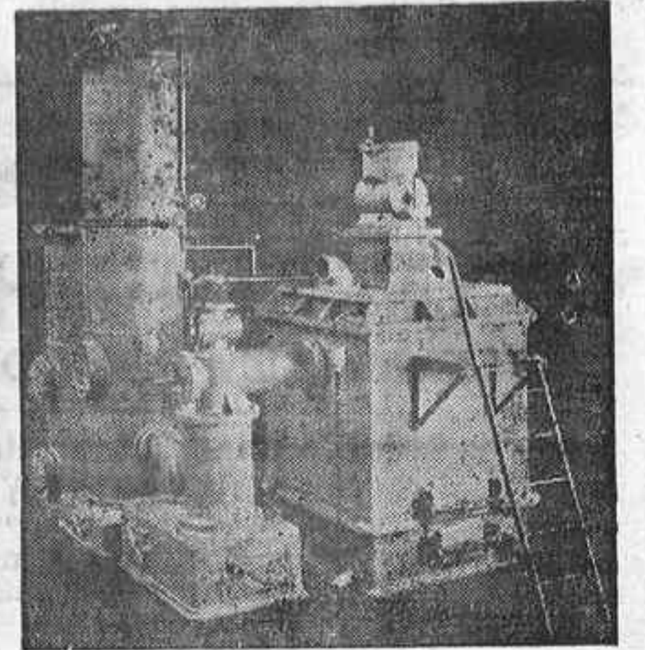
Gasógeno sencillo
