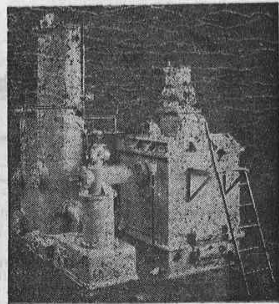
Gasógeno sencillo
