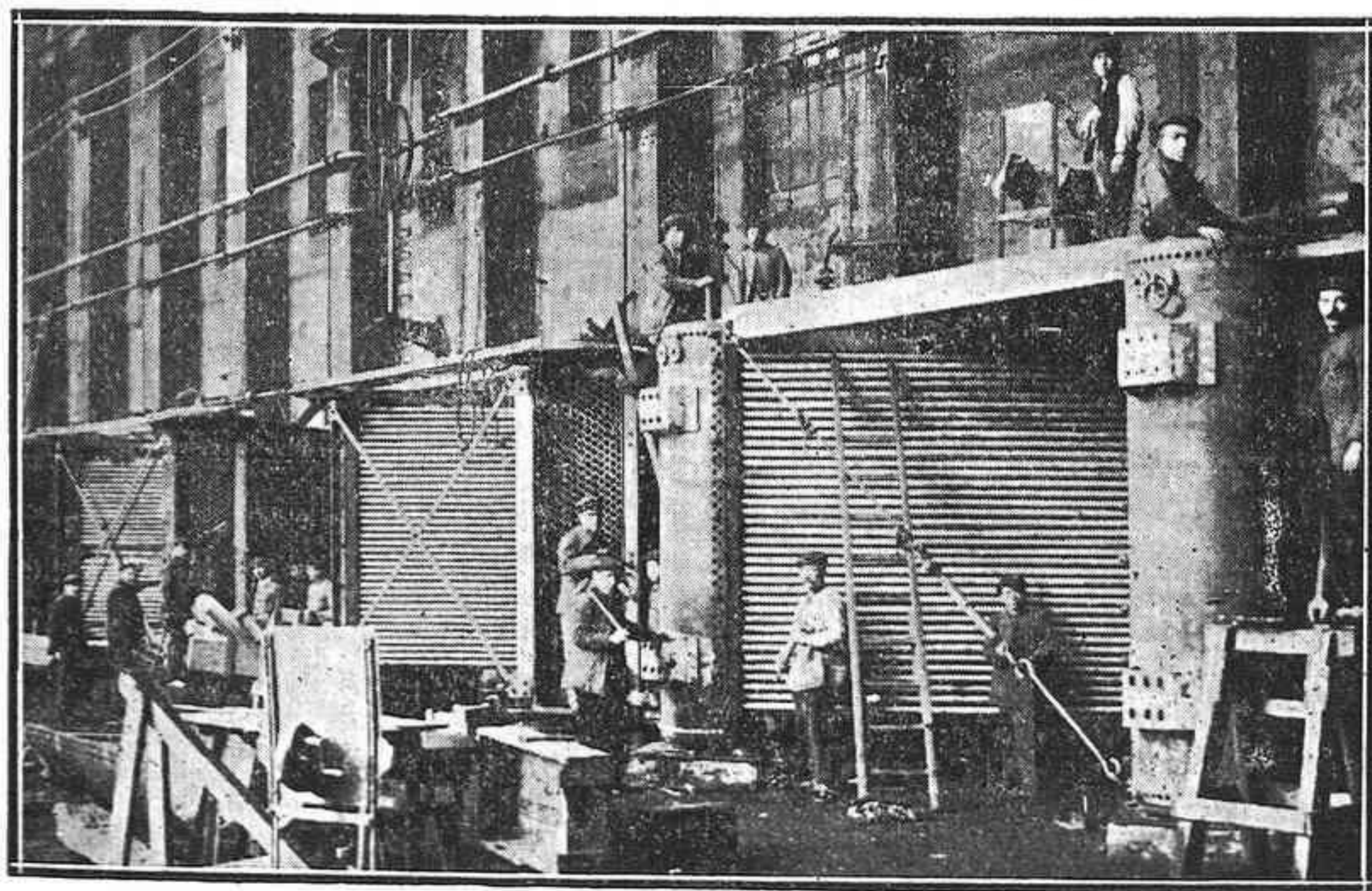
BARCELONA: Calderas del acorazado "España", que se están construyendo en los talleres de "La Maquinista terrestre y marítima"
