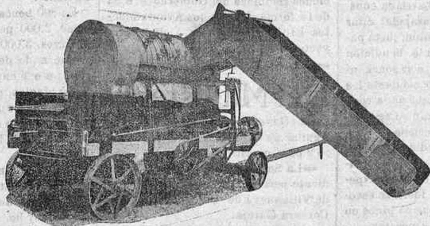
Trilladora HELIAKS-SCHLAYER
