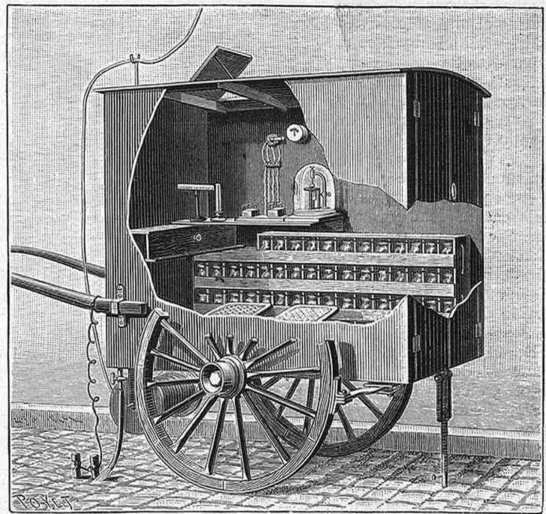
Nuevo laboratorio ambulante para el ensayo de los cables eléctricos
