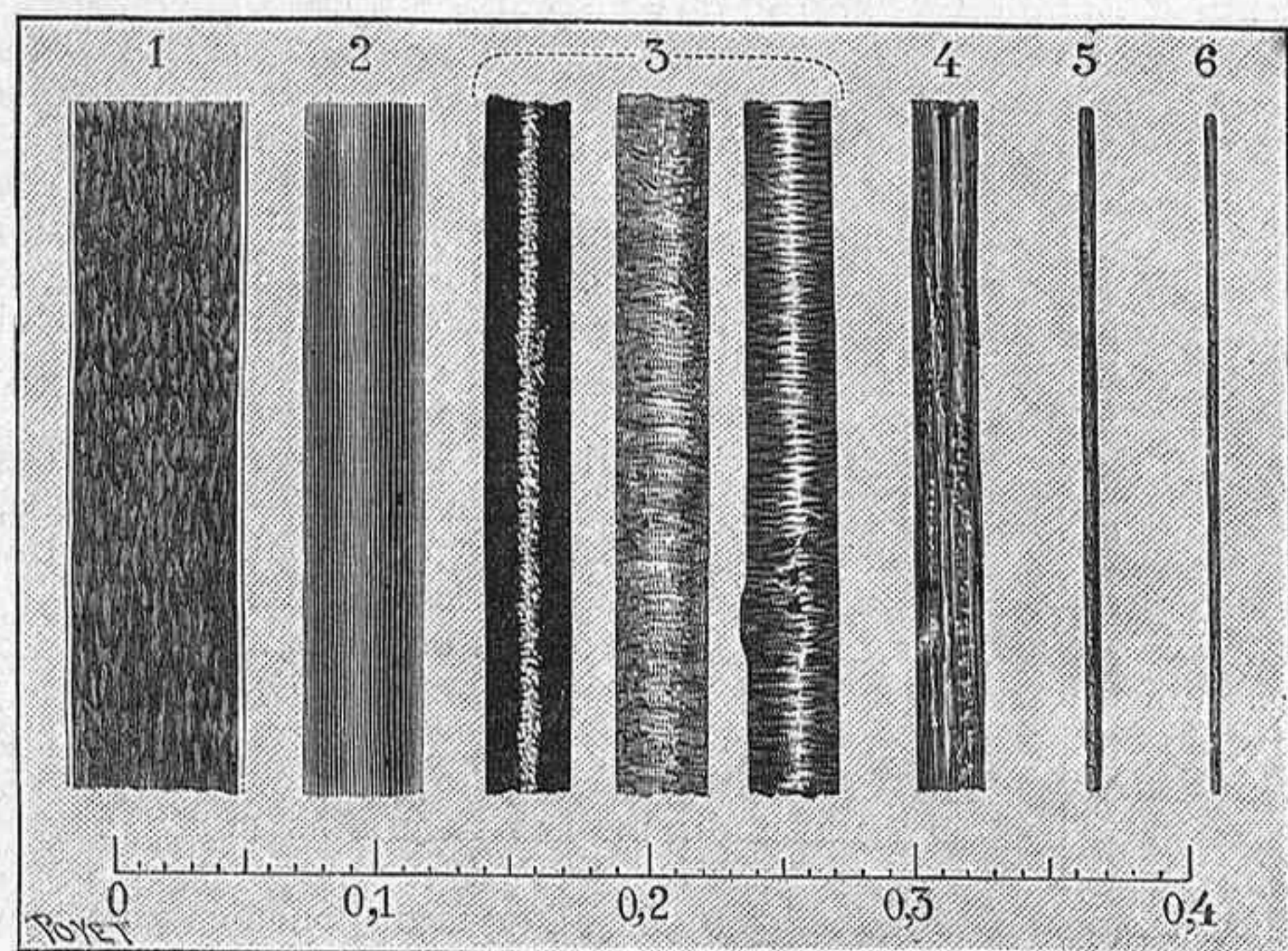
Fibras que pueden servir al establecimiento de suspensiones unifilares. - 1. Cabello fino. - 2. Hilo de cobre. - 3. Hilo de cristal. - 4. Hilo de capullo de seda. - 5 y 6. Hilos de cuarzo. (La escala está indicada por milímetros. Cada división elemental representa una centésima de milímetro.)
