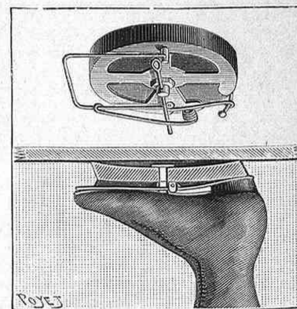
Fig. 2. Detalle del patín neumático
