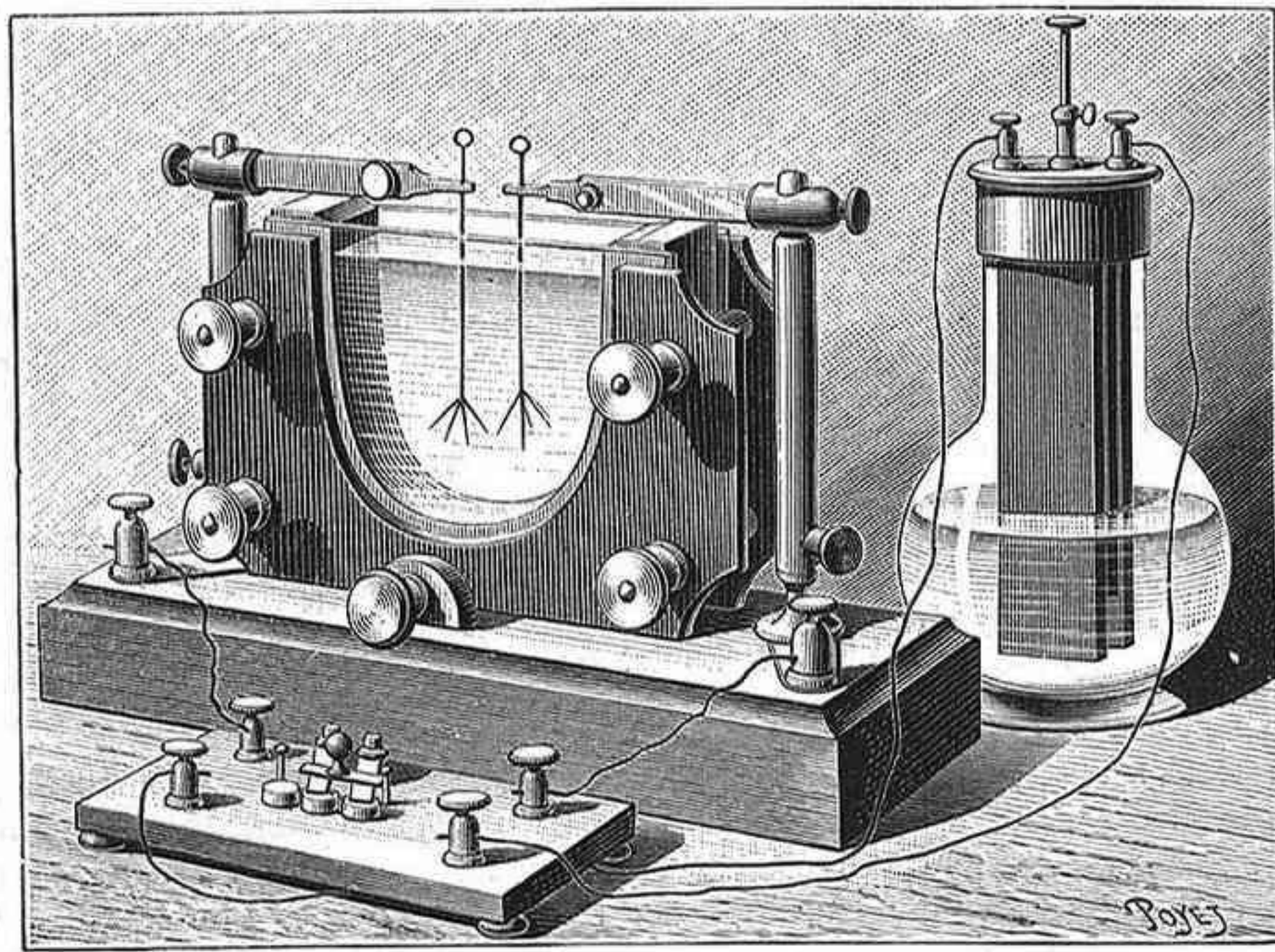
Fig. 1. Cuba-laboratorio para proyecciones
