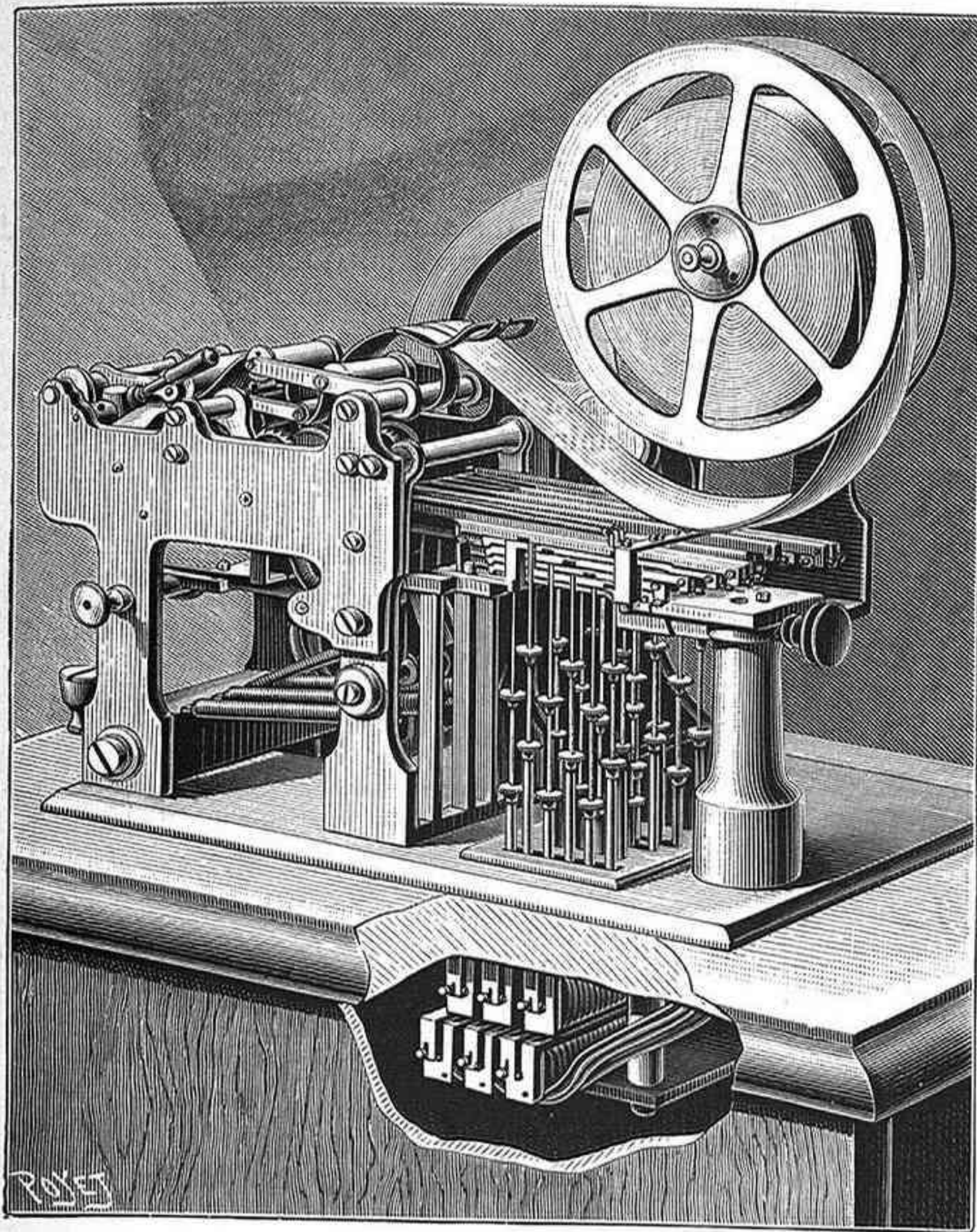
Fig. 1. El telégrafo taquigráfico. Aparato receptor é impresor.
