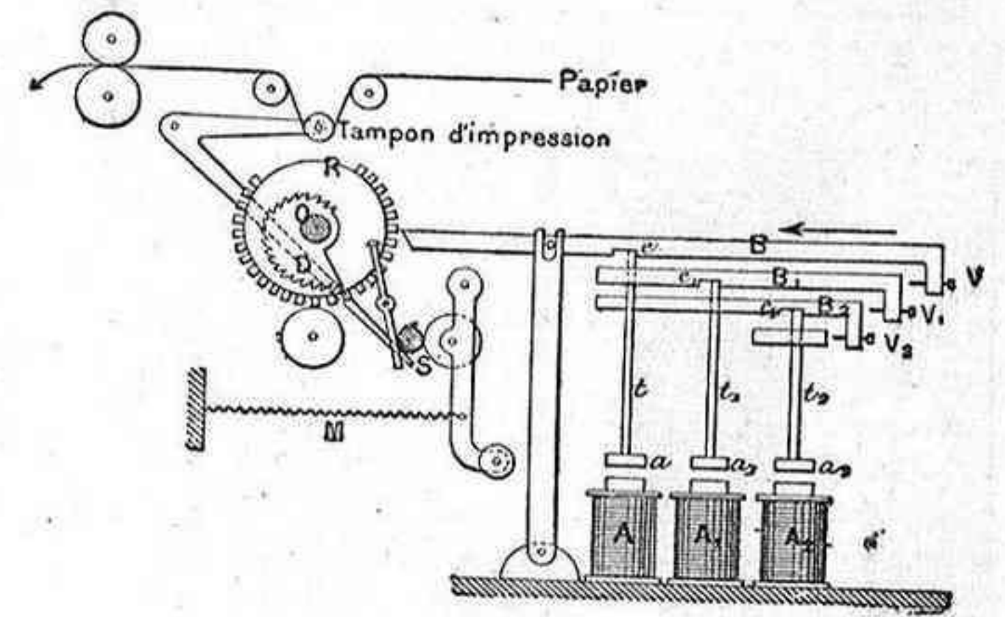
Fig. 2. Diseño del mecanismo del aparato receptor
