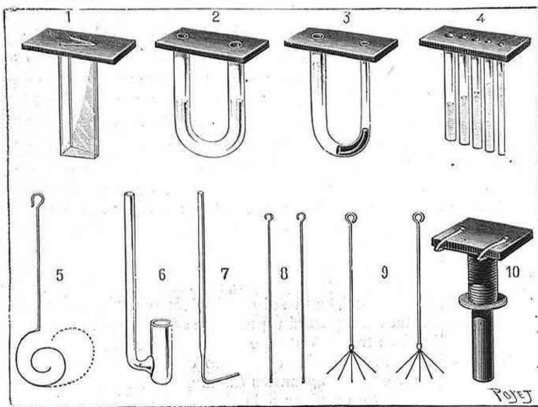
Fig. 3. Accesorios de la cuba-laboratorio para proyecciones
