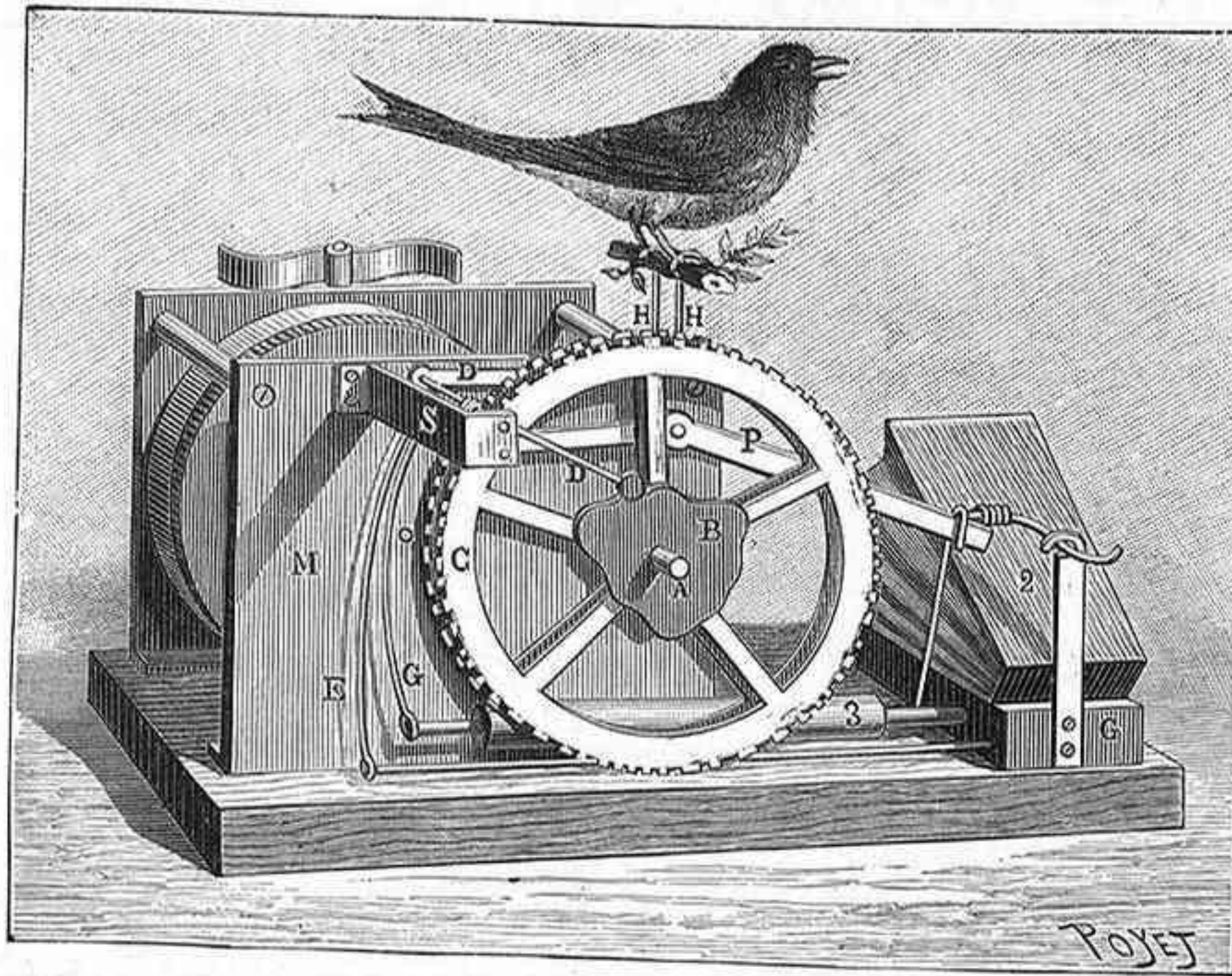
Fig. 5. Mecanismo de un pájaro cantor
