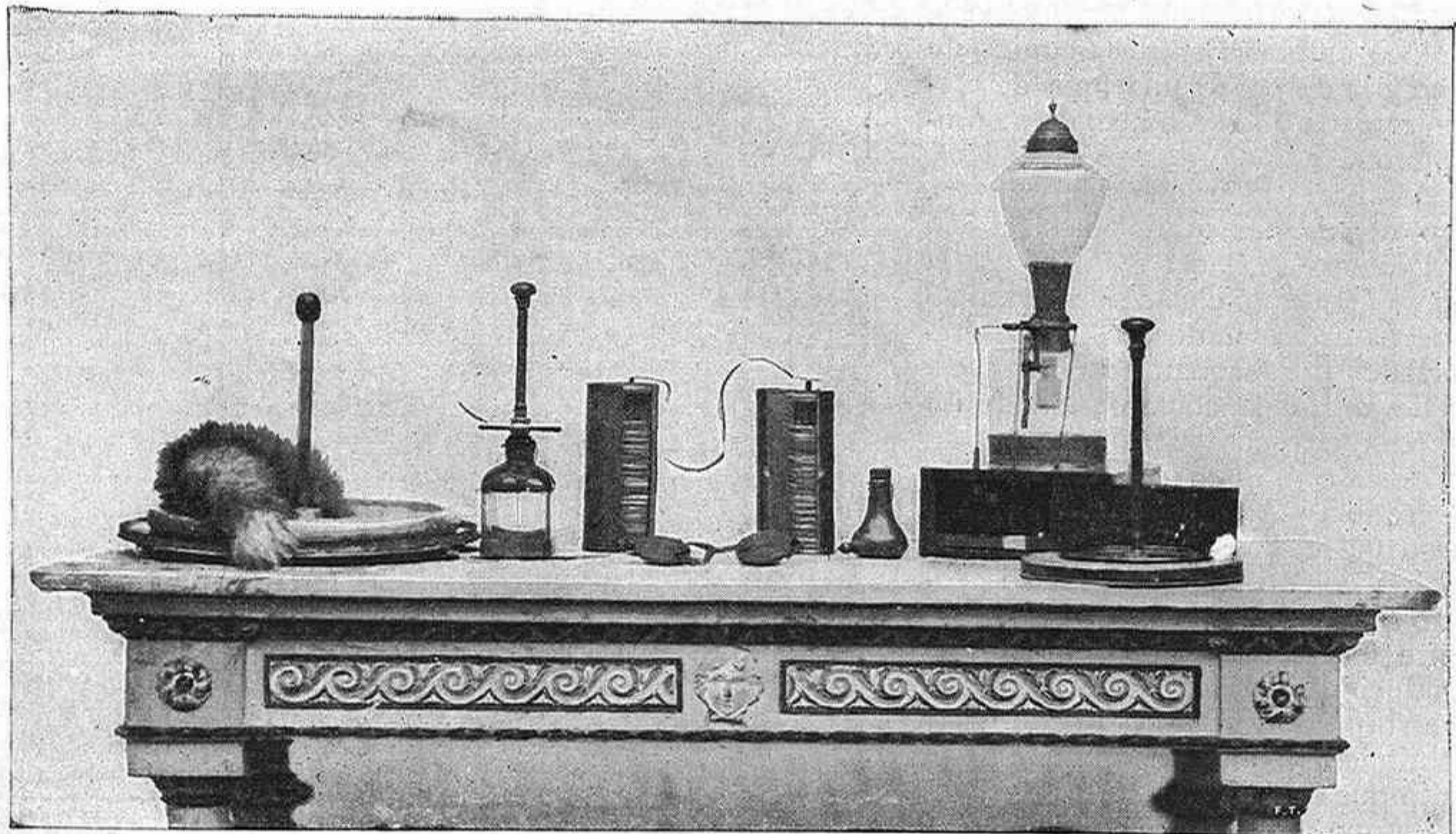
APARATOS DE ALEJANDRO VOLTA QUE SE CONSERVAN EN EL INSTITUTO LOMBARDO DE CIENCIAS DE MILÁN. ELECTRÓFORO. - ELECTRÓMETRO CONDENSADOR. - PILA DE COLUMNA. - PISTOLETE DE VOLTA. - LÁMPARA DE GAS HIDRÓGENO.
