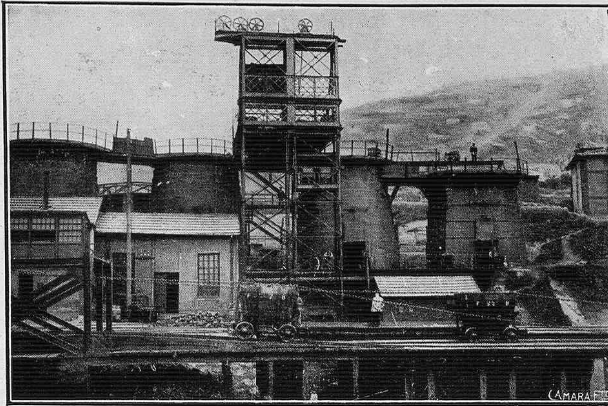
Hornos de calcinación en una mina de Bilbao
