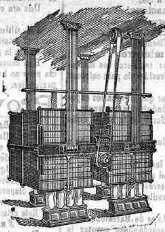
Número planisichter de libre oscilación y equilibrio automático. Privilegio Buhler.
