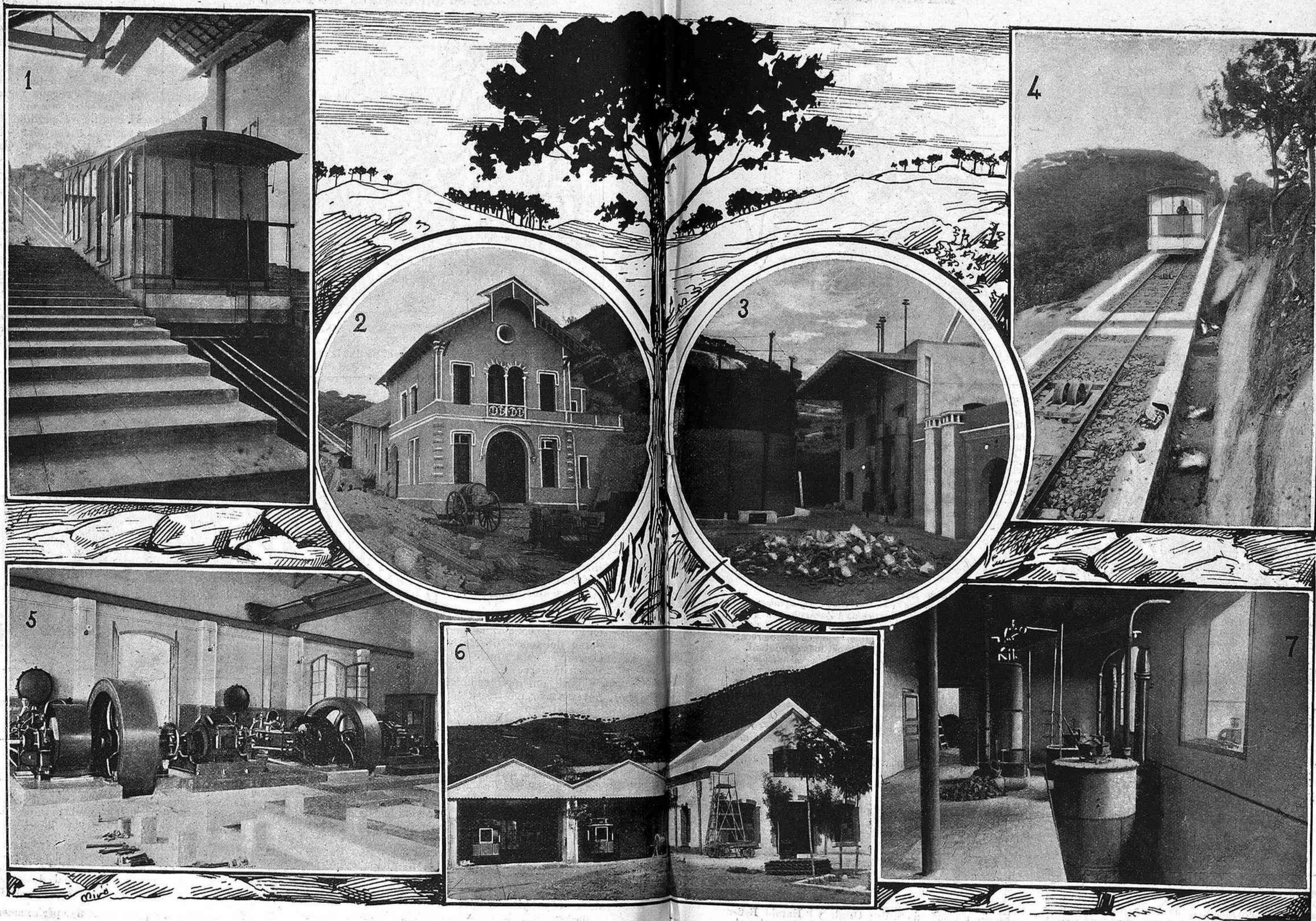
1. Interior de la Estació de sortida.—2. Vista general de la Estació de sortida.—3. Instal·lació dels gasògens Dowson per a la producció del gas pobre.—4. La línia. Un cotxe en moviment.—5. Sala de màquines.—6. Exterior de la Sala de màquines y Dipòsit de cotxes.—7. Calderas de gas pobre.
