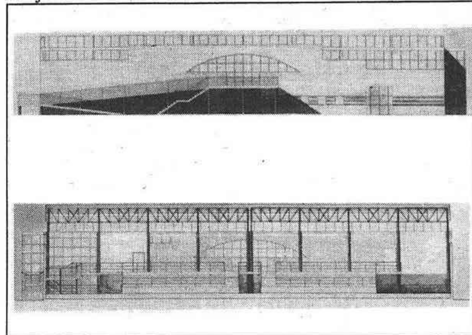
Alzado y sección longitudinal del proyecto de polideportivo que se va a construir en Brihuega, Mondejar y Cifuentes
