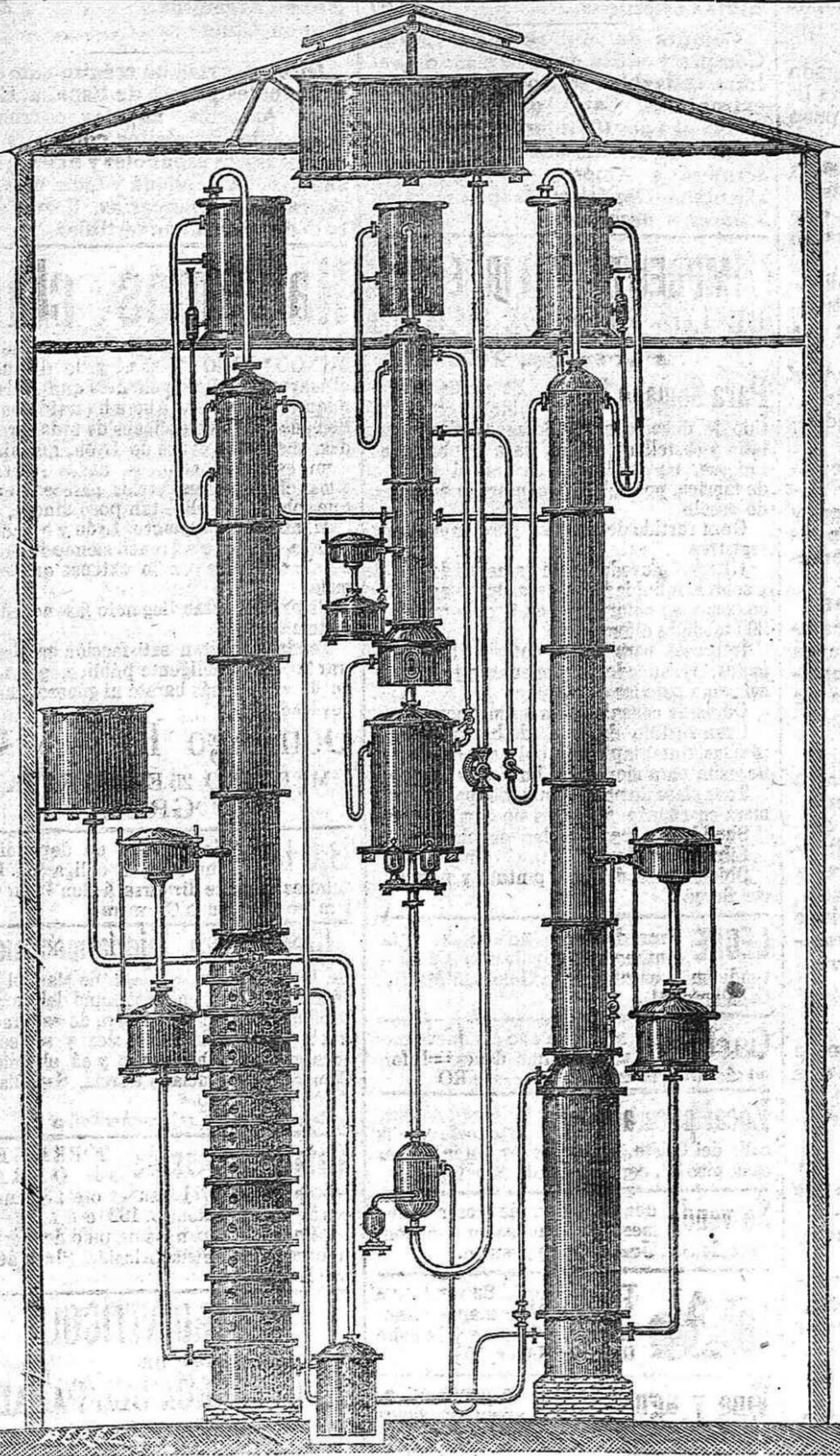
RECTIFICADOR AUTOMÁTICO CONTINUO
