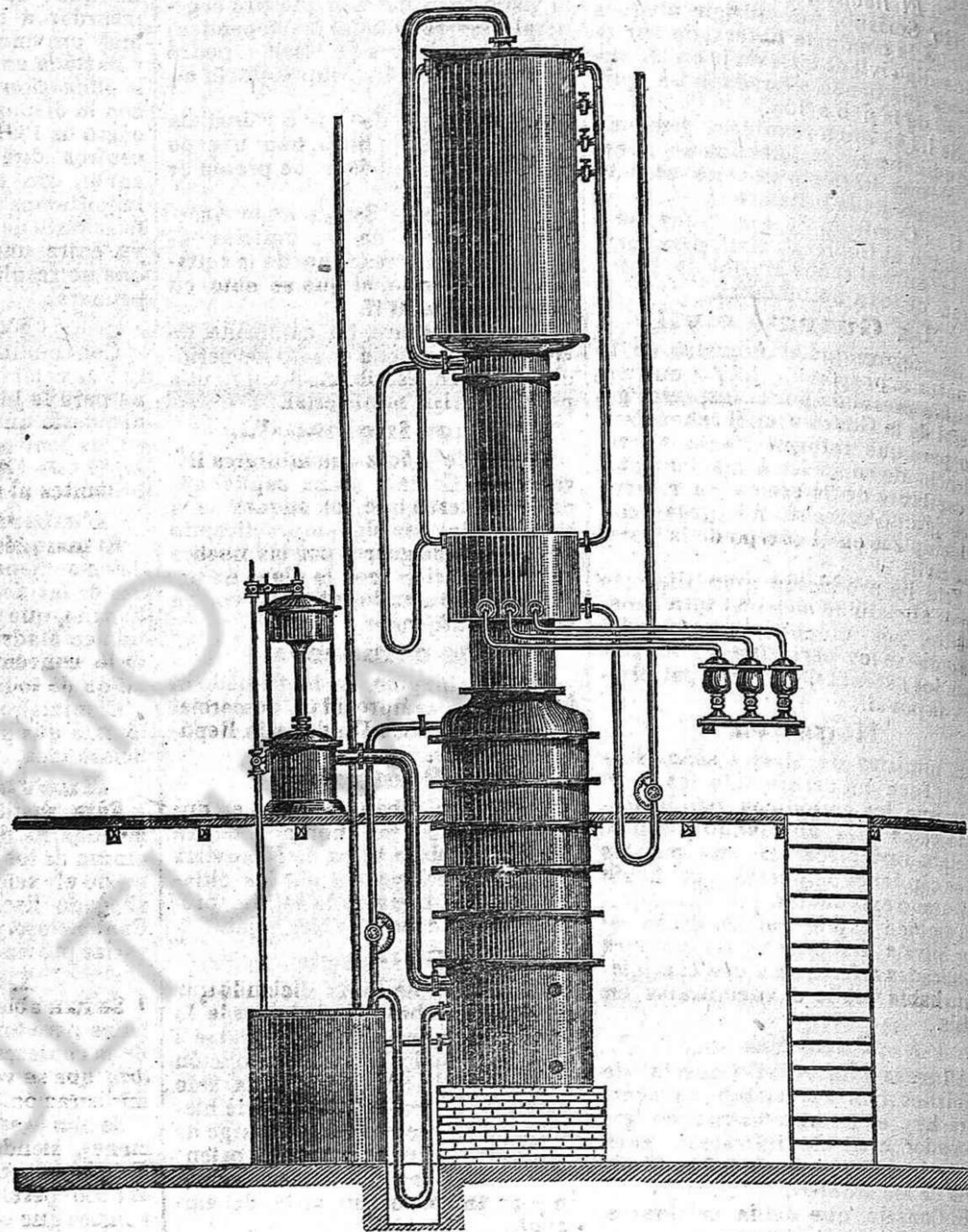
DESTILADOR DEPURADOR CONTINUO O DISCONTINUO
