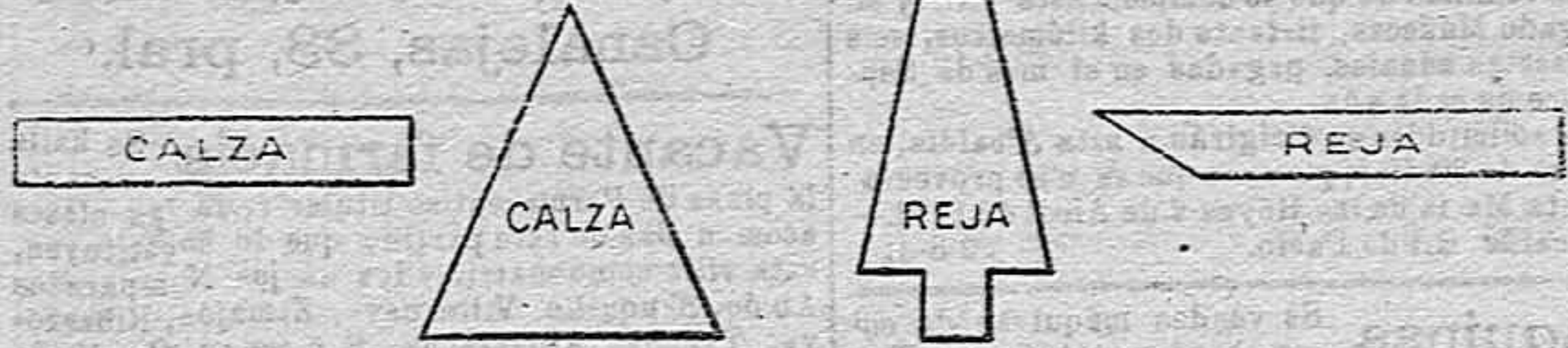
RECORTES Y PLETINAS PARA FABRICACIÓN DE HERRADURAS.
