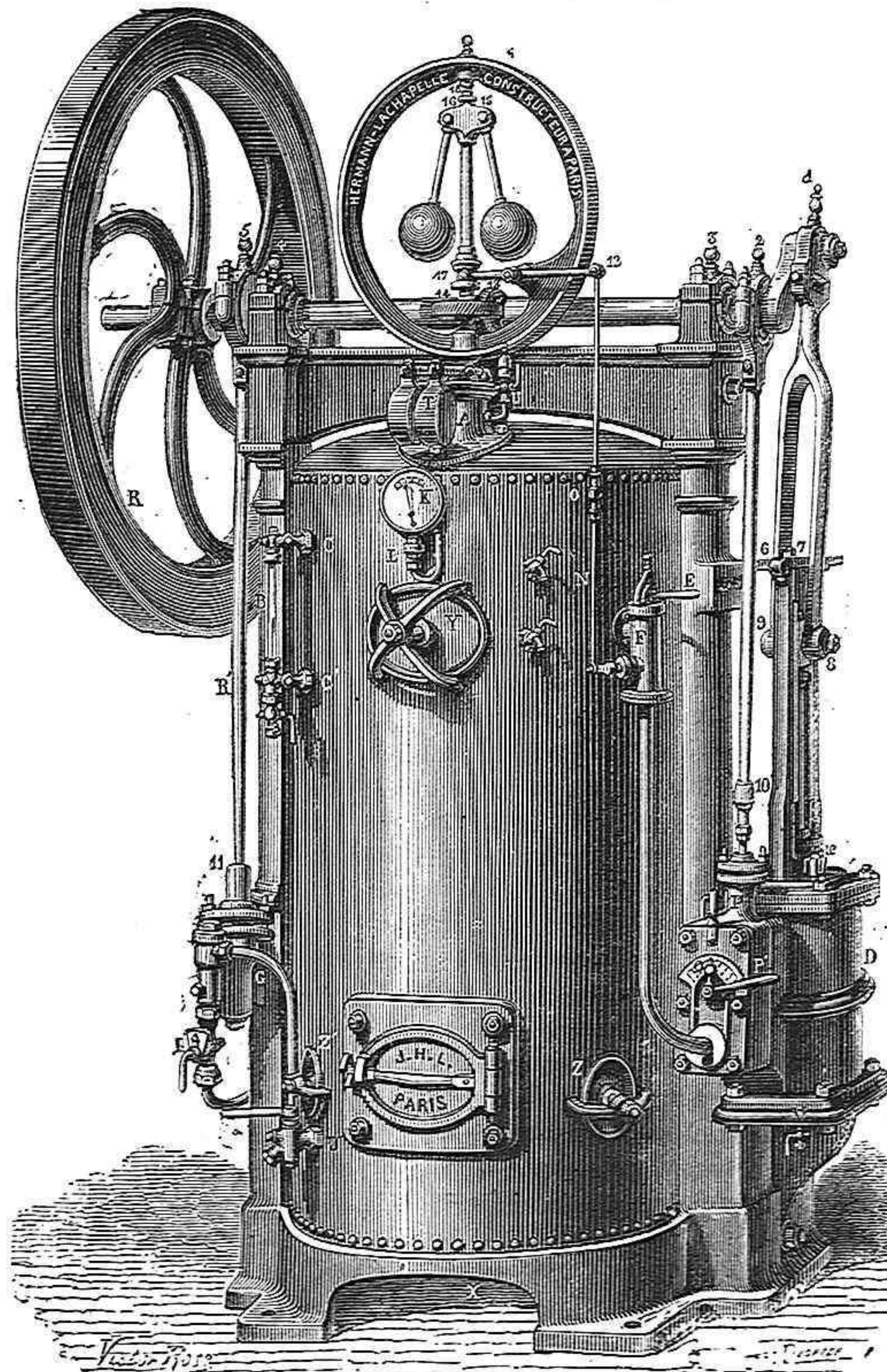
MÁQUINA DE VAPOR, VERTICAL, DE LA CASA J. HERMANN-LACHAPELLE.
