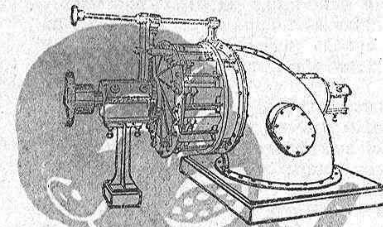
Turbina horizontal "Lefel".
